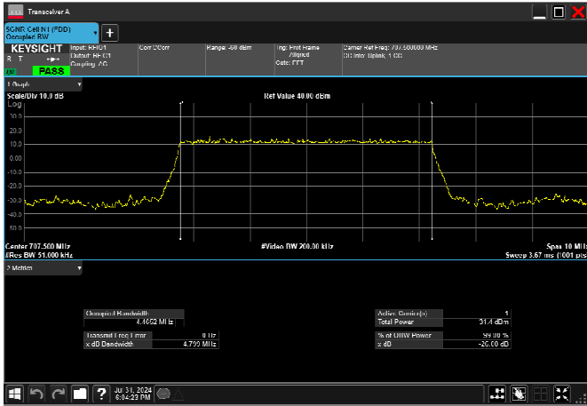
n12_5MHz_15kHz_707.5MHz_DFT-s-OFDM 16 QAM_RB25@0 4.465MHz
