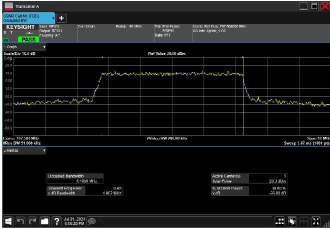
n12_5MHz_15kHz_707.5MHz_CP-OFDM 256 QAM_RB25@0 4.466MHz
