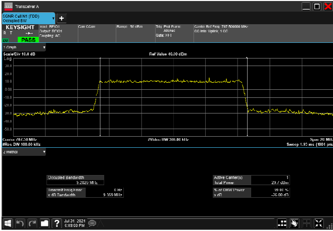
n12_10MHz_15kHz_707.5MHz_CP-OFDM QPSK_RB52@0 9.259MHz
