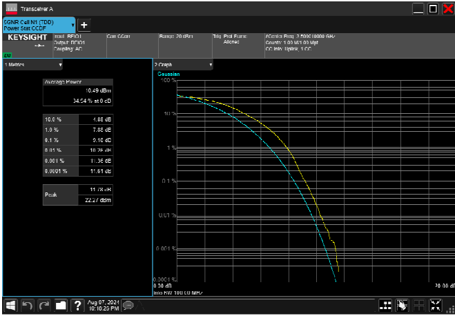
n78_1_100MHz_30kHz_3500MHz_CP-OFDM QPSK_RB273@0 11dB
