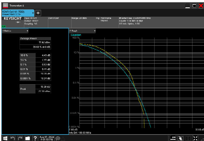
n77_1_100MHz_30kHz_3500MHz_DFT-s-OFDM QPSK_RB270@0 8.63dB
