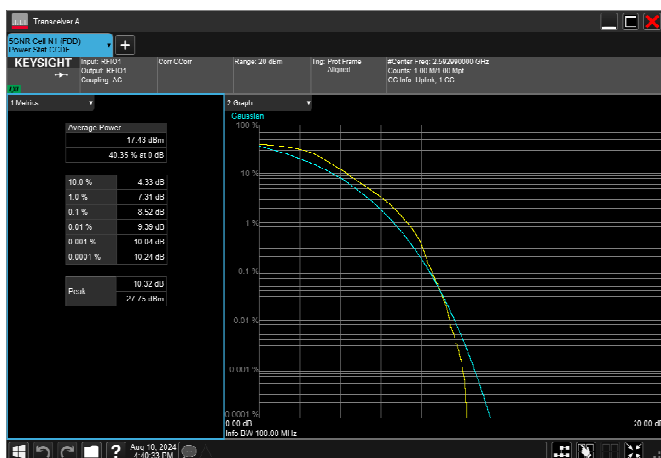
n41_100MHz_30kHz_2592.99MHz_DFT-s-OFDM QPSK_RB270@0 8.52dB
