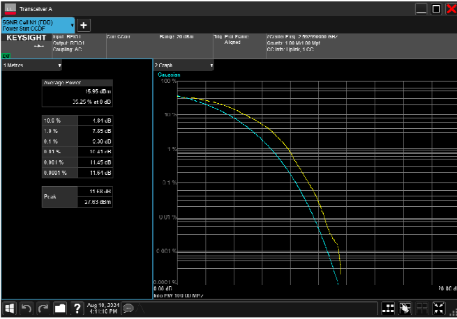
n41_100MHz_30kHz_2592.99MHz_CP-OFDM QPSK_RB273@0 11.15dB
