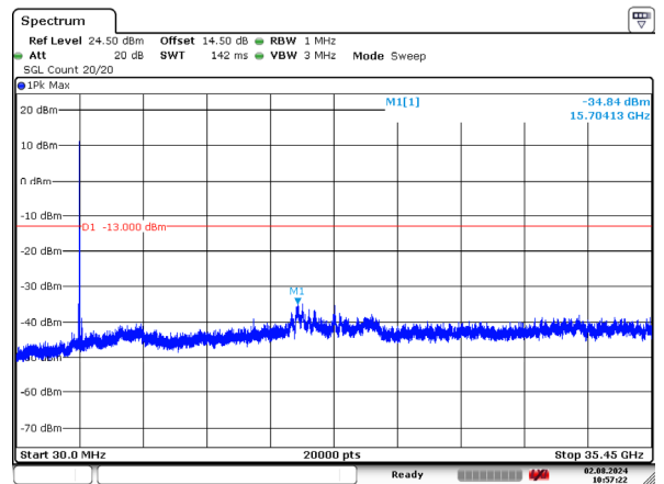
1_10MHz_High_QPSK_50@0 -34.84dBm
