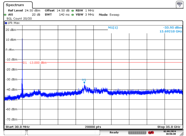
1_10MHz_Middle_QPSK_50@0 -33.95dBm
