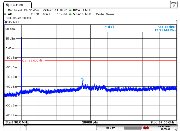
1_10MHz_Low_QPSK_50@0 -35.38dBm
