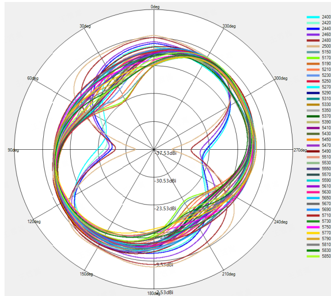
BT/WIFI-2.4G & 5G Phi=0deg
