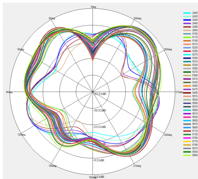
BT/WIFI-2.4G & 5G Theta=90deg
