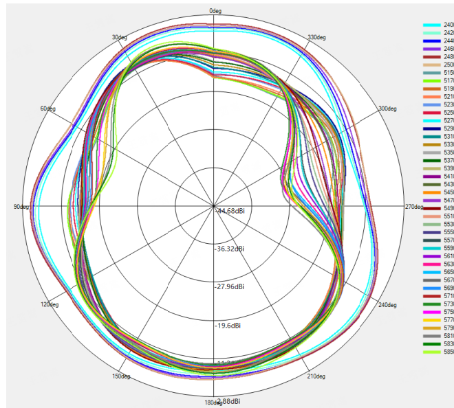
BT/WIFI-2.4G & 5G Phi=90deg
