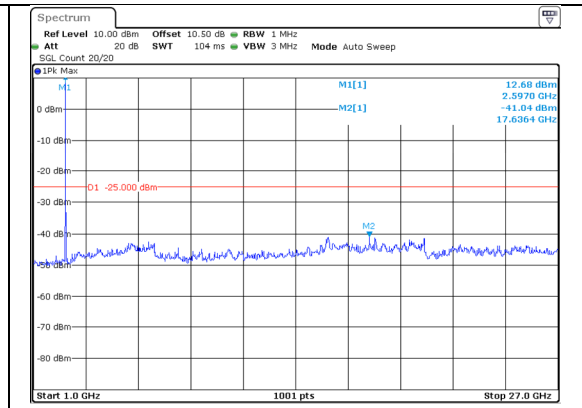
1000.0MHz-27000.0MHz Band 41 20MHz/2590.5/Mid QPSK 1@99 Band 41 5MHz/2602.2/Mid QPSK 1@0
