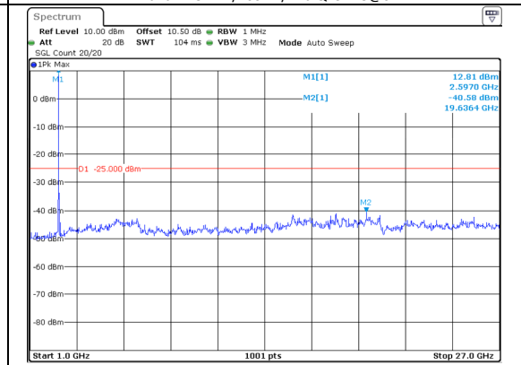
1000.0MHz-27000.0MHz Band 41 20MHz/2590.5/Mid QPSK 100@0 Band 41 5MHz/2602.2/Mid QPSK 25@0
