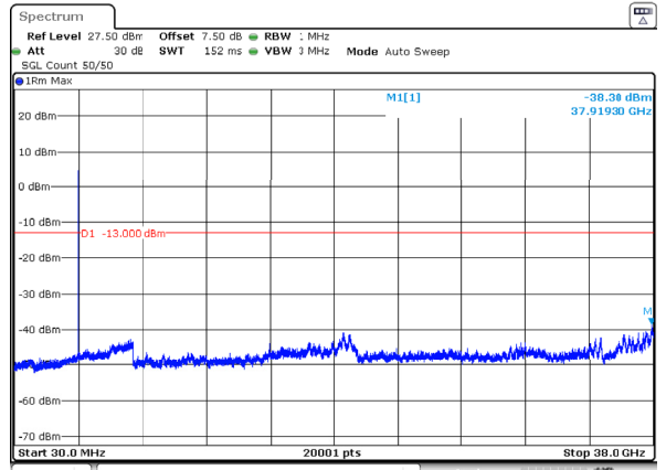
n78_3_20MHz_30kHz_3790MHz_DFT-s-OFDM QPSK_RB50@0 -38.30dBm
