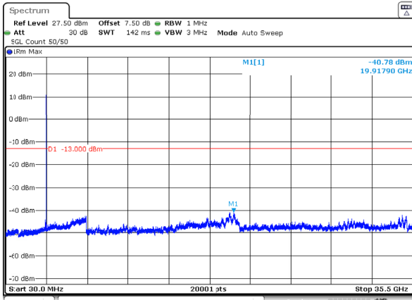
n78_1_90MHz_30kHz_3495MHz_DFT-s-OFDM QPSK_RB1@244 -40.78dBm
