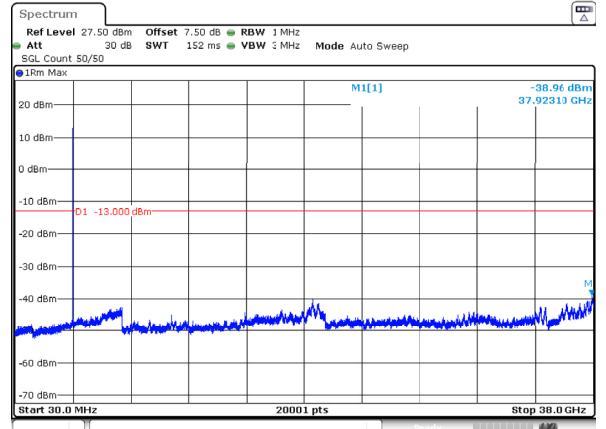
n78_3_30MHz_30kHz_3785MHz_DFT-s-OFDM QPSK_RB1@77 -38.96dBm
