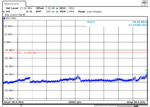
n78_3_10MHz_30kHz_3795MHz_DFT-s-OFDM QPSK_RB24@0 -38.68dBm
