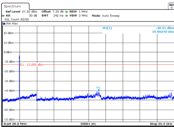
n78_1_90MHz_30kHz_3500MHz_DFT-s-OFDM QPSK_RB243@0 -40.51dBm
