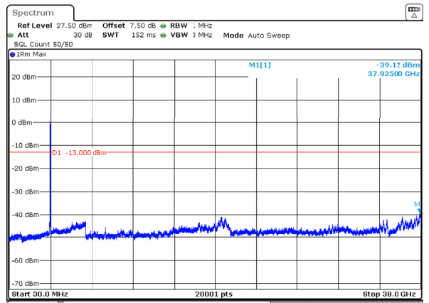
n78_3_50MHz_30kHz_3750MHz_DFT-s-OFDM QPSK_RB128@0 -39.12dBm
