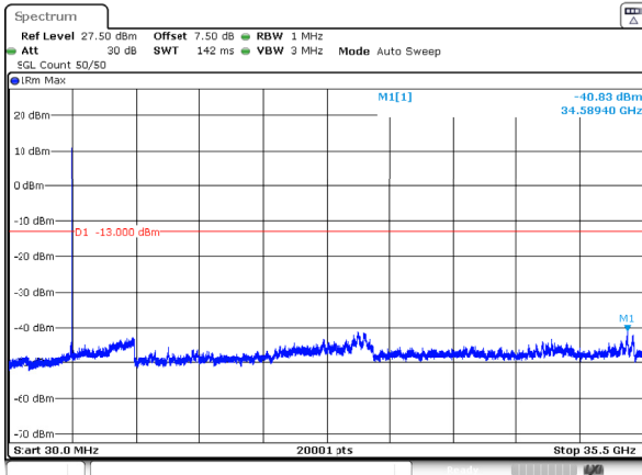
n78_1_90MHz_30kHz_3505MHz_DFT-s-OFDM QPSK_RB1@244 -40.83dBm
