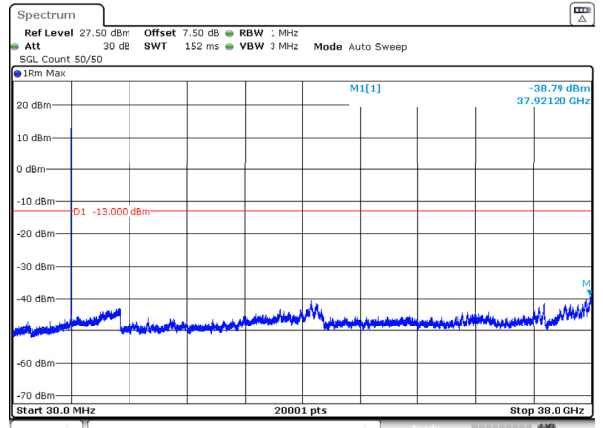
n78_3_40MHz_30kHz_3780MHz_DFT-s-OFDM QPSK_RB1@105 -38.79dBm
