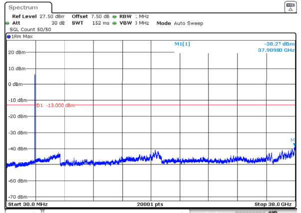
n78_3_10MHz_30kHz_3705MHz_DFT-s-OFDM QPSK_RB24@0 -38.27dBm
