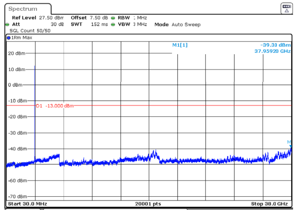
n78_3_30MHz_30kHz_3750MHz_DFT-s-OFDM QPSK_RB1@0 -39.33dBm
