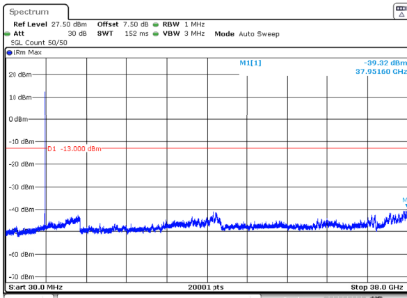
n78_3_20MHz_30kHz_3710MHz_DFT-s-OFDM QPSK_RB1@50 -39.32dBm
