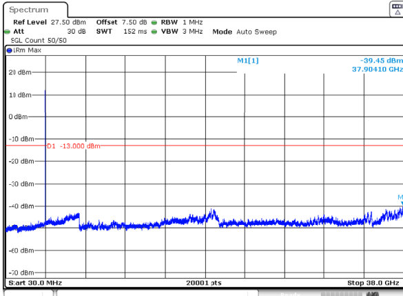
n78_3_15MHz_30kHz_3792.5MHz_DFT-s-OFDM QPSK_RB1@0 -39.45dBm
