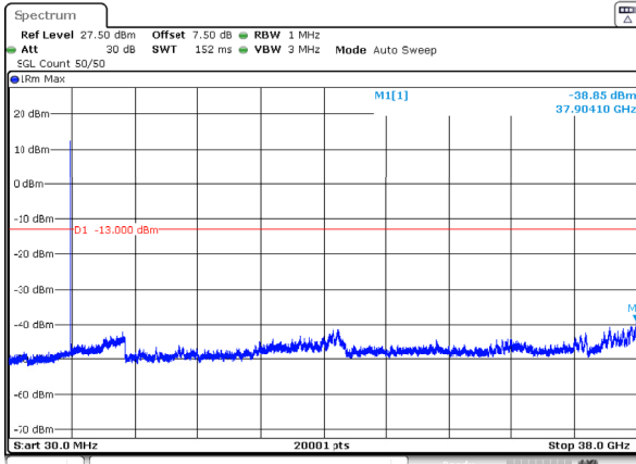
n78_3_10MHz_30kHz_3750MHz_DFT-s-OFDM QPSK_RB1@0 -38.85dBm
