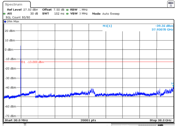
n78_3_15MHz_30kHz_3750MHz_DFT-s-OFDM QPSK_RB36@0 -39.35dBm
