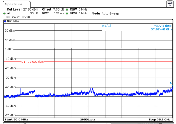
n78_3_50MHz_30kHz_3725MHz_DFT-s-OFDM QPSK_RB1@0 -39.40dBm
