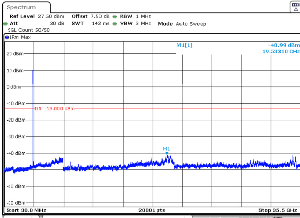
n78_1_90MHz_30kHz_3500MHz_DFT-s-OFDM QPSK_RB1@0 -40.99dBm
