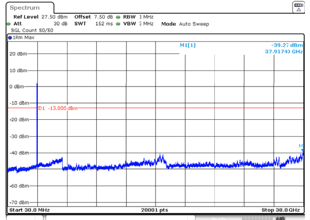
n78_3_30MHz_30kHz_3750MHz_DFT-s-OFDM QPSK_RB75@0 -39.27dBm
