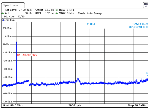
n78_3_20MHz_30kHz_3750MHz_DFT-s-OFDM QPSK_RB50@0 -39.14dBm
