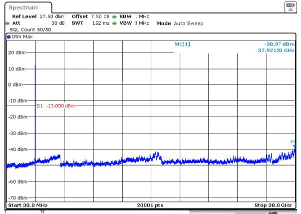
n78_3_40MHz_30kHz_3720MHz_DFT-s-OFDM QPSK_RB1@105 -38.97dBm
