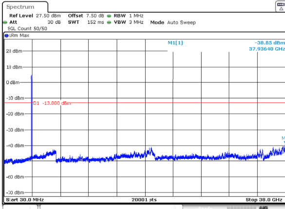
n78_3_15MHz_30kHz_3707.5MHz_DFT-s-OFDM QPSK_RB1@0 -38.85dBm
