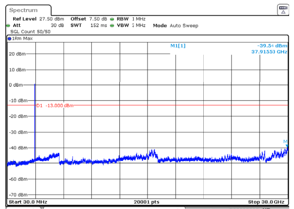
n78_3_40MHz_30kHz_3720MHz_DFT-s-OFDM QPSK_RB100@0 -39.54dBm
