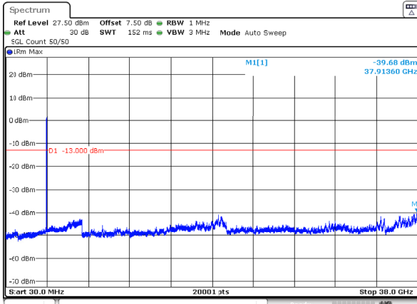
n78_3_40MHz_30kHz_3750MHz_DFT-s-OFDM QPSK_RB100@0 -39.68dBm
