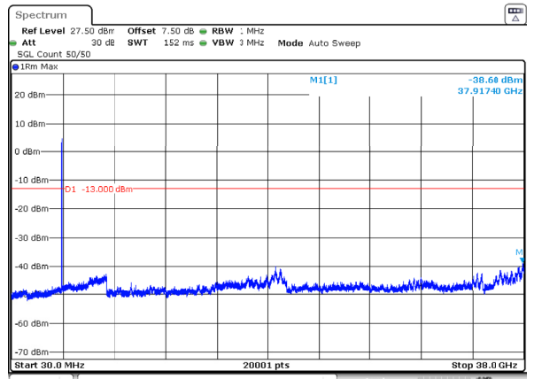
n78_3_20MHz_30kHz_3710MHz_DFT-s-OFDM QPSK_RB50@0 -38.60dBm
