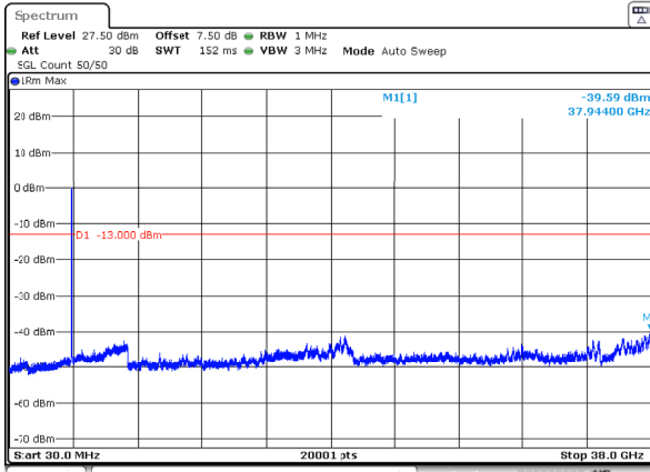
n78_3_50MHz_30kHz_3725MHz_DFT-s-OFDM QPSK_RB128@0 -39.59dBm
