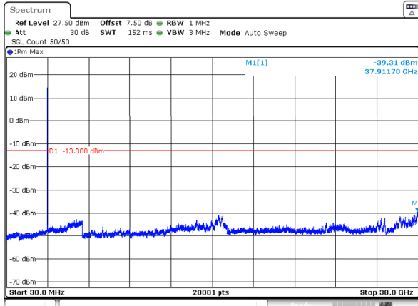
n78_3_30MHz_30kHz_3785MHz_DFT-s-OFDM QPSK_RB1@0 -39.31dBm
