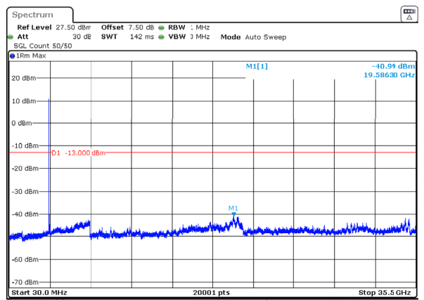
n78_1_90MHz_30kHz_3505MHz_DFT-s-OFDM QPSK_RB1@0 -40.99dBm
