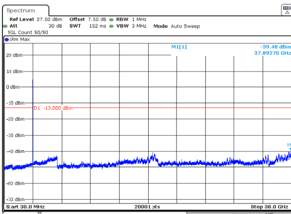
n78_3_15MHz_30kHz_3792.5MHz_DFT-s-OFDM QPSK_RB36@0 -39.48dBm
