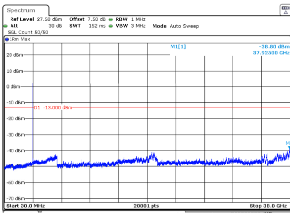
n78_3_30MHz_30kHz_3785MHz_DFT-s-OFDM QPSK_RB75@0 -38.80dBm
