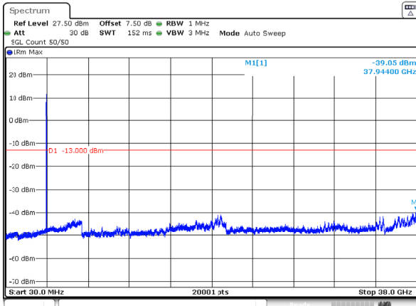
n78_3_15MHz_30kHz_3750MHz_DFT-s-OFDM QPSK_RB1@37 -39.05dBm
