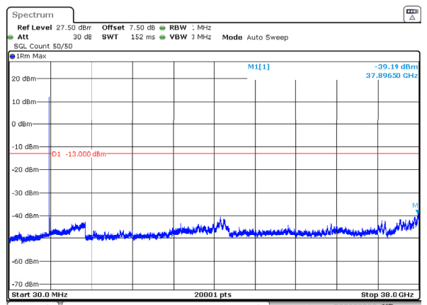
n78_3_20MHz_30kHz_3710MHz_DFT-s-OFDM QPSK_RB1@0 -39.19dBm
