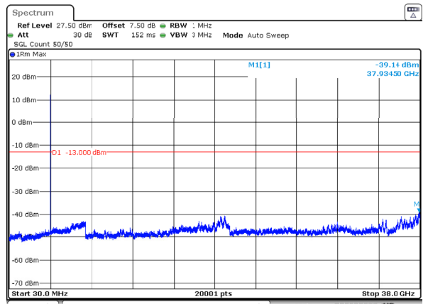
n78_3_10MHz_30kHz_3795MHz_DFT-s-OFDM QPSK_RB1@0 -39.14dBm
