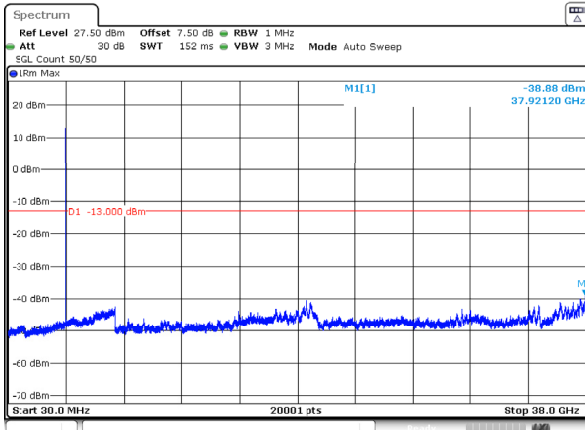
n78_3_10MHz_30kHz_3795MHz_DFT-s-OFDM QPSK_RB1@23 -38.88dBm
