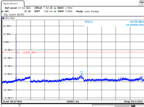
n78_1_100MHz_30kHz_3500MHz_DFT-s-OFDM QPSK_RB1@0 -40.98dBm
