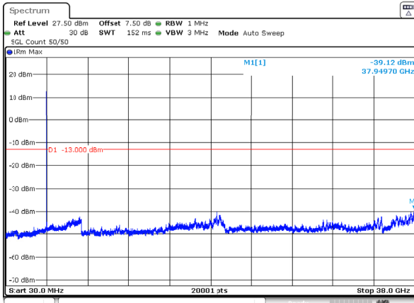
n78_3_40MHz_30kHz_3780MHz_DFT-s-OFDM QPSK_RB1@0 -39.12dBm
