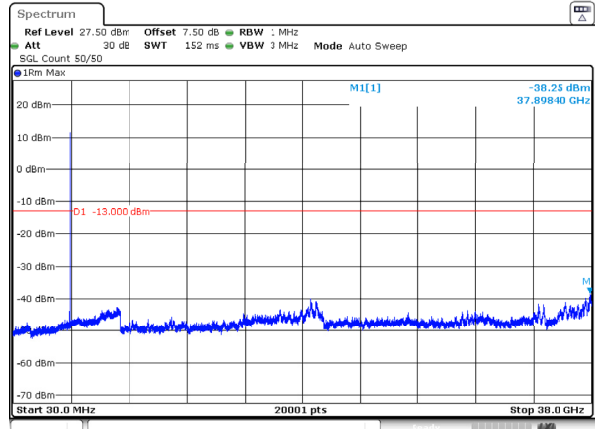
n78_3_15MHz_30kHz_3707.5MHz_DFT-s-OFDM QPSK_RB1@37 -38.25dBm
