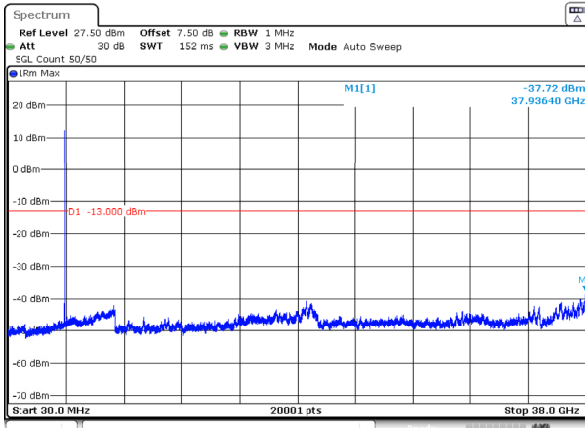
n78_3_10MHz_30kHz_3705MHz_DFT-s-OFDM QPSK_RB1@23 -37.72dBm
