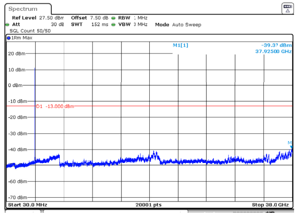
n78_3_15MHz_30kHz_3750MHz_DFT-s-OFDM QPSK_RB1@0 -39.37dBm
