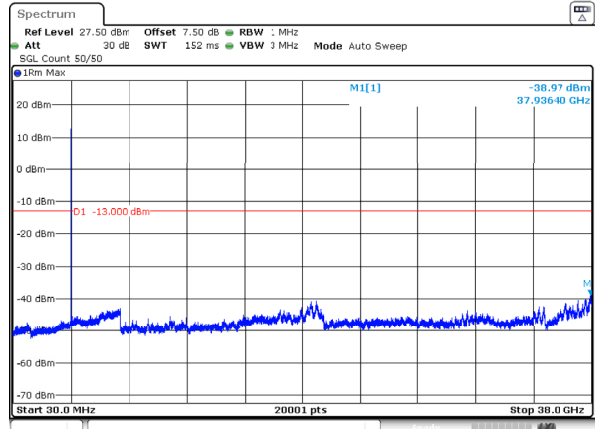
n78_3_15MHz_30kHz_3792.5MHz_DFT-s-OFDM QPSK_RB1@37 -38.97dBm
