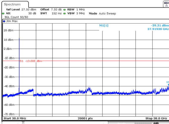
n78_3_30MHz_30kHz_3750MHz_DFT-s-OFDM QPSK_RB1@77 -39.31dBm
