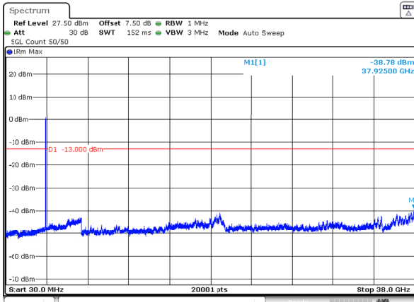
n78_3_40MHz_30kHz_3720MHz_DFT-s-OFDM QPSK_RB1@0 -38.78dBm
