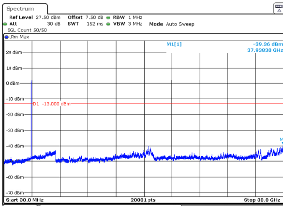
n78_3_30MHz_30kHz_3715MHz_DFT-s-OFDM QPSK_RB75@0 -39.36dBm
