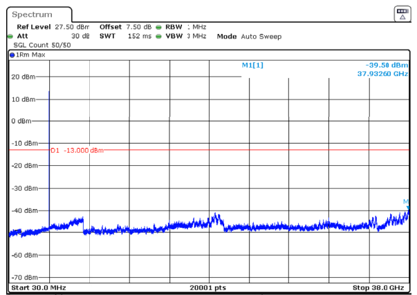
n78_3_20MHz_30kHz_3790MHz_DFT-s-OFDM QPSK_RB1@0 -39.50dBm
