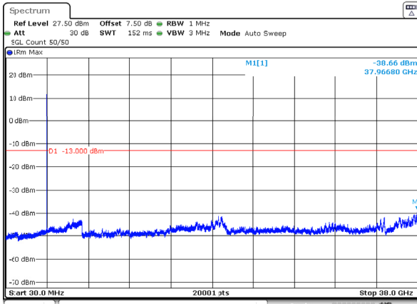
n78_3_20MHz_30kHz_3790MHz_DFT-s-OFDM QPSK_RB1@50 -38.66dBm
