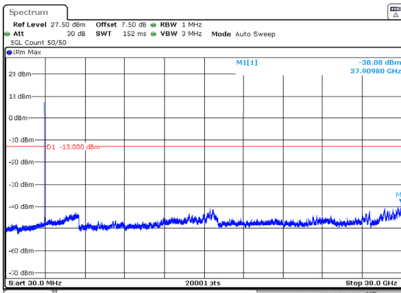
n78_3_10MHz_30kHz_3750MHz_DFT-s-OFDM QPSK_RB24@0 -38.08dBm
