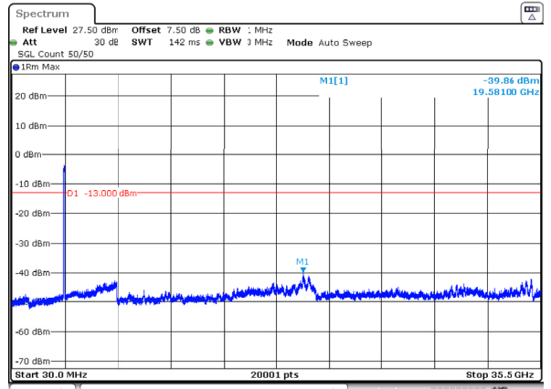
n78_1_90MHz_30kHz_3495MHz_DFT-s-OFDM QPSK_RB243@0 -39.86dBm
