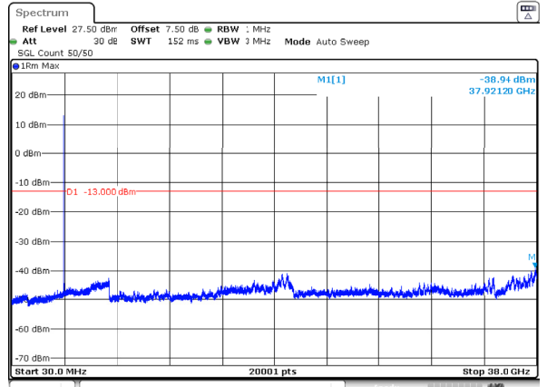
n78_3_40MHz_30kHz_3750MHz_DFT-s-OFDM QPSK_RB1@0 -38.94dBm
