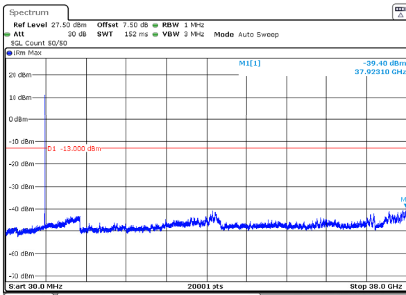
n78_3_50MHz_30kHz_3725MHz_DFT-s-OFDM QPSK_RB1@132 -39.40dBm
