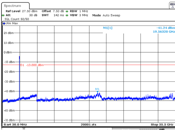
n78_1_100MHz_30kHz_3500MHz_DFT-s-OFDM QPSK_RB270@0 -41.24dBm
