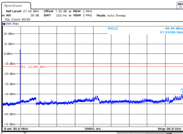
n78_3_15MHz_30kHz_3707.5MHz_DFT-s-OFDM QPSK_RB36@0 -38.99dBm
