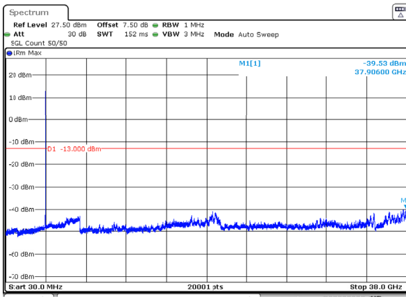
n78_3_40MHz_30kHz_3750MHz_DFT-s-OFDM QPSK_RB1@105 -39.53dBm
