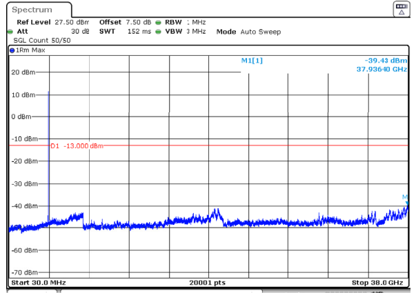
n78_3_30MHz_30kHz_3715MHz_DFT-s-OFDM QPSK_RB1@77 -39.43dBm
