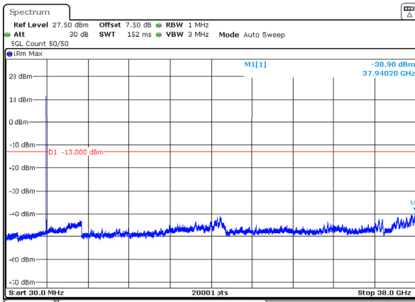
n78_3_20MHz_30kHz_3750MHz_DFT-s-OFDM QPSK_RB1@0 -38.90dBm
