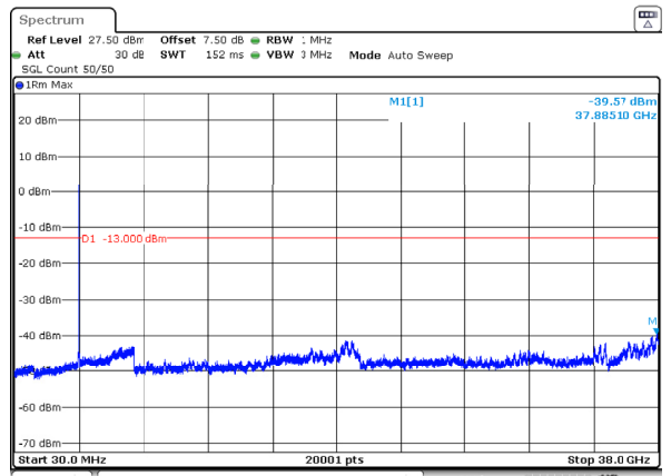
n78_3_40MHz_30kHz_3780MHz_DFT-s-OFDM QPSK_RB100@0 -39.57dBm
