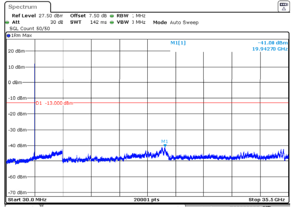
n78_1_90MHz_30kHz_3500MHz_DFT-s-OFDM QPSK_RB1@244 -41dBm
