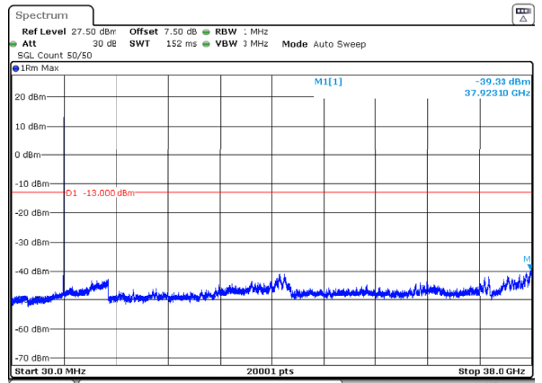
n78_3_20MHz_30kHz_3750MHz_DFT-s-OFDM QPSK_RB1@50 -39.33dBm
