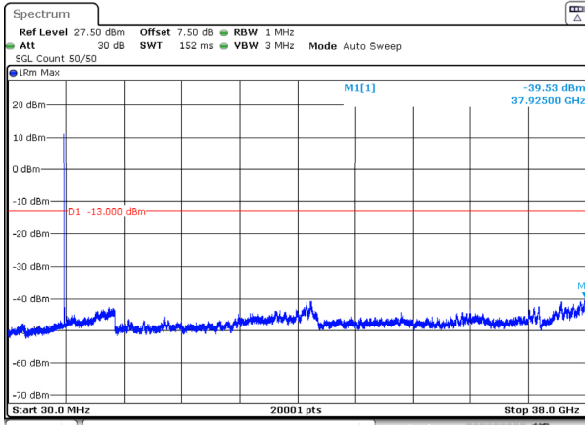
n78_3_30MHz_30kHz_3715MHz_DFT-s-OFDM QPSK_RB1@0 -39.53dBm
