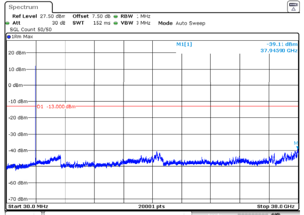
n78_3_10MHz_30kHz_3750MHz_DFT-s-OFDM QPSK_RB1@23 -39.11dBm
