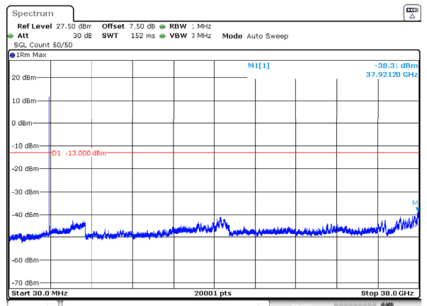
n78_3_10MHz_30kHz_3705MHz_DFT-s-OFDM QPSK_RB1@0 -38.31dBm
