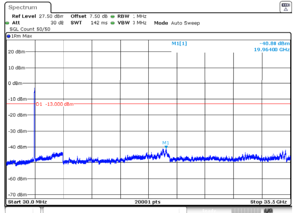
n78_1_90MHz_30kHz_3505MHz_DFT-s-OFDM QPSK_RB243@0 -40.80dBm
