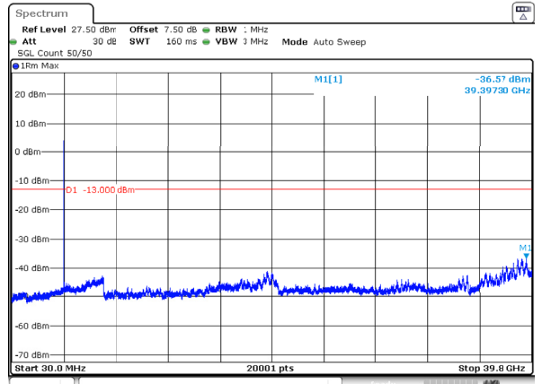
n77_3_20MHz_30kHz_3970MHz_DFT-s-OFDM QPSK_RB50@0 -36.57dBm
