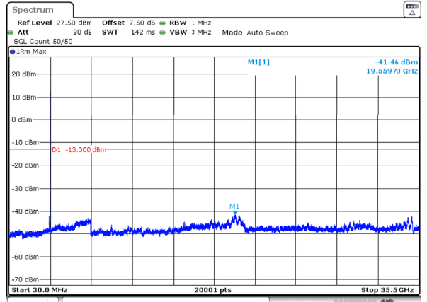
n77_1_90MHz_30kHz_3500MHz_DFT-s-OFDM QPSK_RB1@244 -41.46dBm
