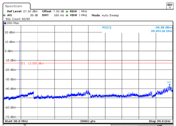
n77_3_20MHz_30kHz_3710MHz_DFT-s-OFDM QPSK_RB1@0 -36.88dBm
