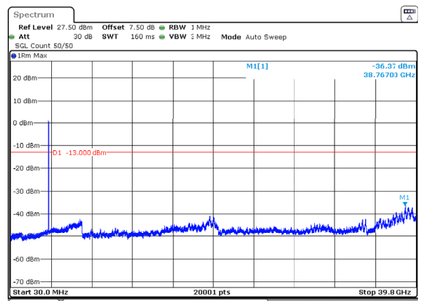
n77_3_40MHz_30kHz_3720MHz_DFT-s-OFDM QPSK_RB100@0 -36.37dBm
