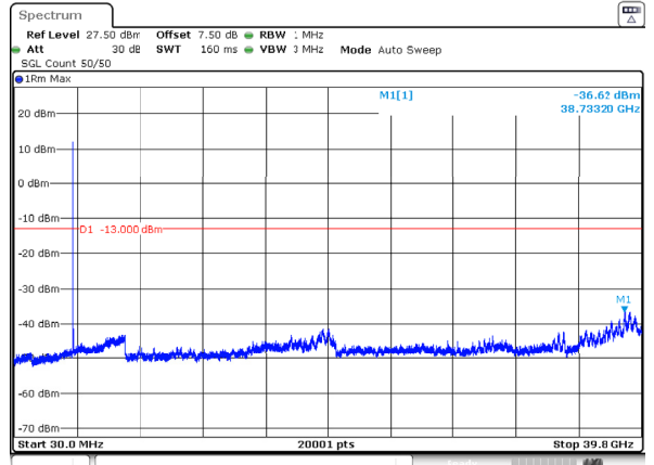
n77_3_50MHz_30kHz_3725MHz_DFT-s-OFDM QPSK_RB1@0 -36.62dBm
