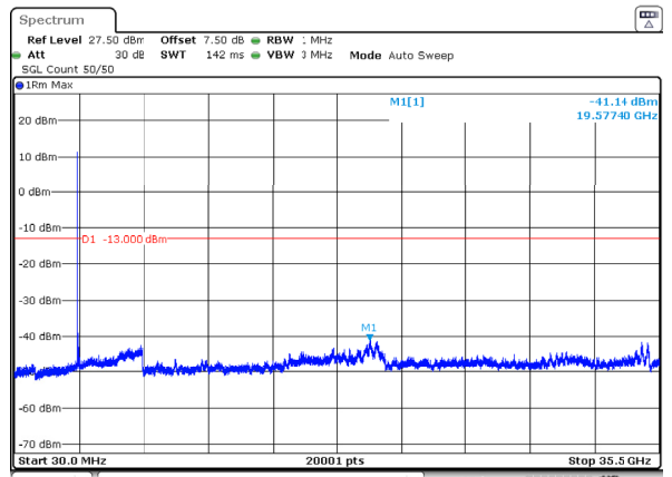
n77_1_90MHz_30kHz_3505MHz_DFT-s-OFDM QPSK_RB1@0 -41.14dBm
