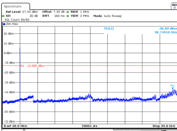
n77_3_15MHz_30kHz_3972.5MHz_DFT-s-OFDM QPSK_RB36@0 -36.85dBm
