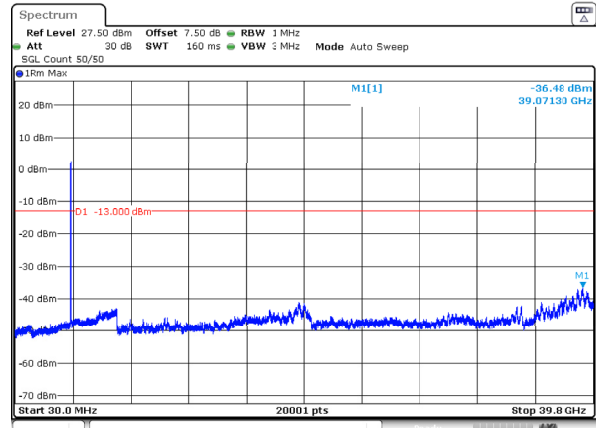
n77_3_30MHz_30kHz_3840MHz_DFT-s-OFDM QPSK_RB75@0 -36.48dBm
