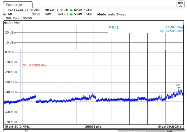
n77_3_20MHz_30kHz_3710MHz_DFT-s-OFDM QPSK_RB50@0 -36.58dBm
