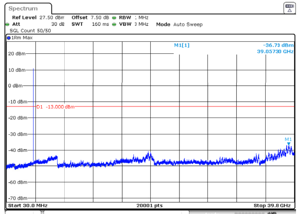
n77_3_15MHz_30kHz_3707.5MHz_DFT-s-OFDM QPSK_RB1@37 -36.73dBm
