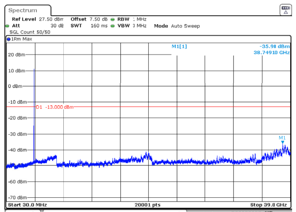
n77_3_15MHz_30kHz_3840MHz_DFT-s-OFDM QPSK_RB1@0 -35.98dBm
