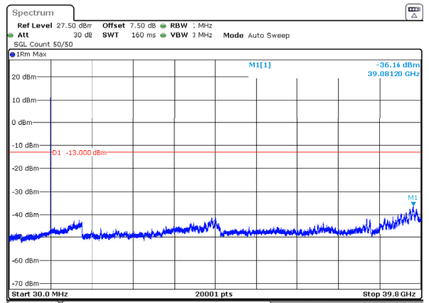
n77_3_10MHz_30kHz_3975MHz_DFT-s-OFDM QPSK_RB1@0 -36.16dBm
