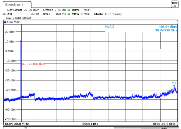
n77_3_40MHz_30kHz_3720MHz_DFT-s-OFDM QPSK_RB1@105 -36.64dBm
