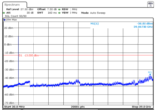
n77_3_20MHz_30kHz_3970MHz_DFT-s-OFDM QPSK_RB1@0 -36.85dBm
