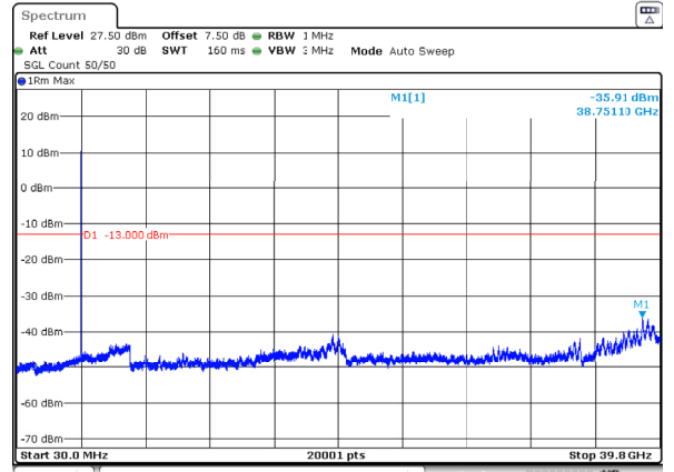
n77_3_30MHz_30kHz_3965MHz_DFT-s-OFDM QPSK_RB1@77 -35.91dBm
