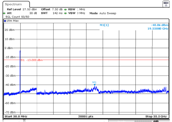
n77_1_90MHz_30kHz_3505MHz_DFT-s-OFDM QPSK_RB243@0 -40.86dBm
