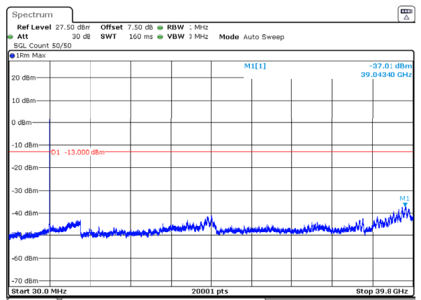
n77_3_40MHz_30kHz_3960MHz_DFT-s-OFDM QPSK_RB100@0 -37.01dBm
