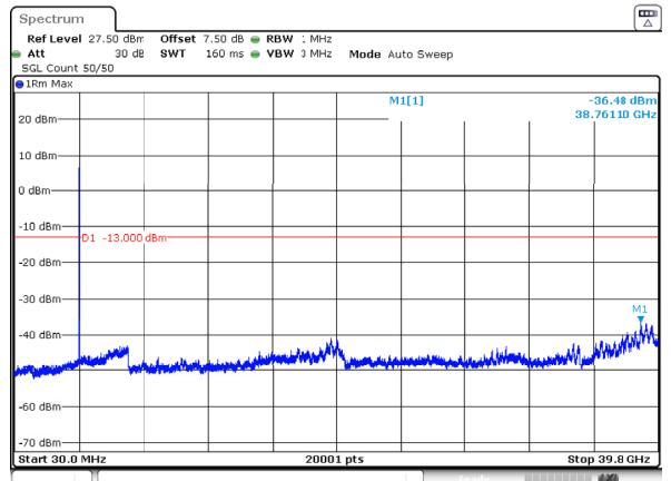
n77_3_10MHz_30kHz_3975MHz_DFT-s-OFDM QPSK_RB24@0 -36.48dBm
