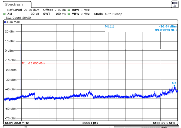
n77_3_10MHz_30kHz_3705MHz_DFT-s-OFDM QPSK_RB24@0 -36.98dBm
