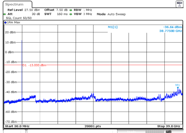
n77_3_15MHz_30kHz_3972.5MHz_DFT-s-OFDM QPSK_RB1@37 -36.66dBm
