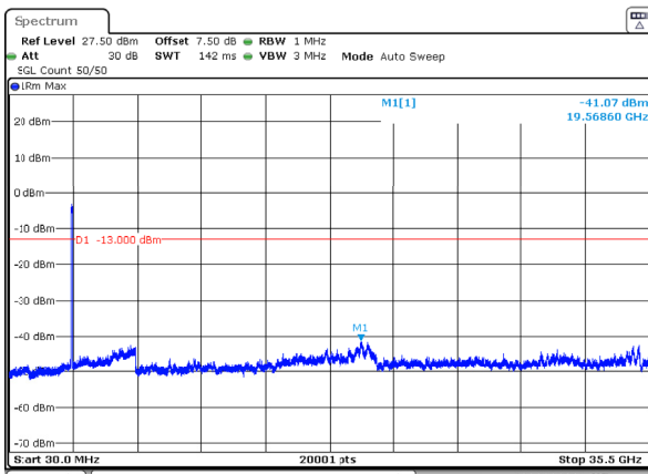
n77_1_100MHz_30kHz_3500MHz_DFT-s-OFDM QPSK_RB270@0 -41.07dBm
