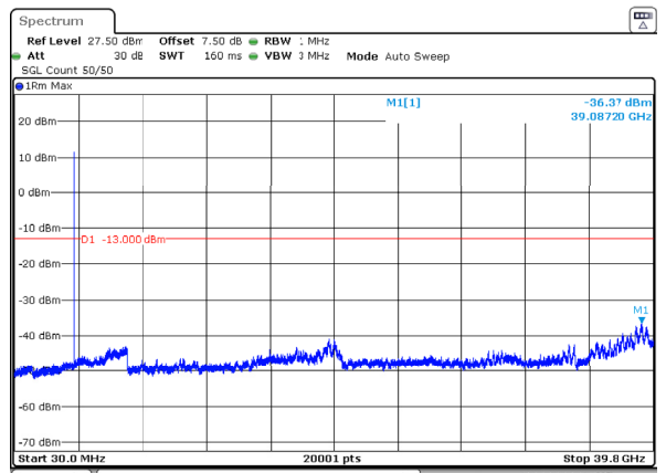
n77_3_10MHz_30kHz_3705MHz_DFT-s-OFDM QPSK_RB1@0 -36.37dBm
