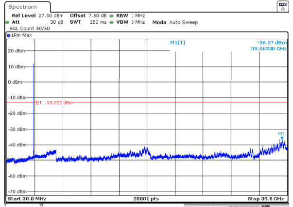
n77_3_40MHz_30kHz_3840MHz_DFT-s-OFDM QPSK_RB1@0 -36.27dBm
