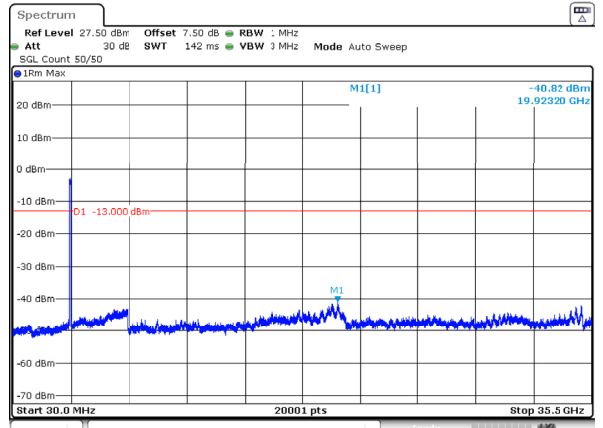
n77_1_90MHz_30kHz_3495MHz_DFT-s-OFDM QPSK_RB243@0 -40.82dBm
