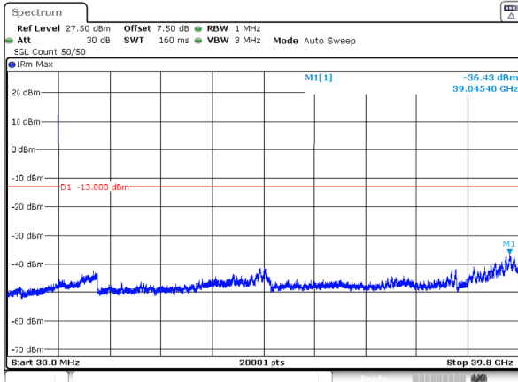
n77_3_15MHz_30kHz_3972.5MHz_DFT-s-OFDM QPSK_RB1@0 -36.43dBm
