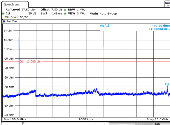
n77_1_60MHz_30kHz_3500MHz_DFT-s-OFDM QPSK_RB1@0 -40.30dBm
