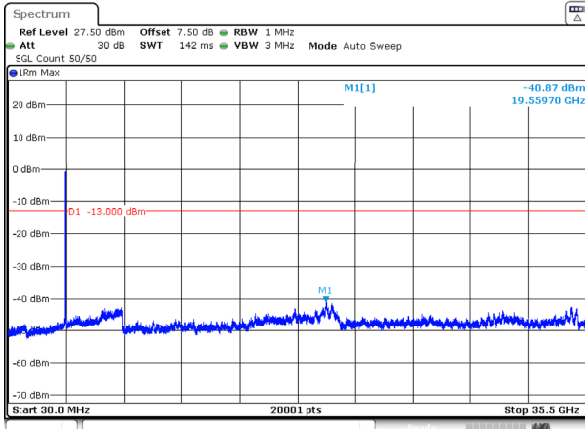
n77_1_60MHz_30kHz_3520MHz_DFT-s-OFDM QPSK_RB162@0 -40.87dBm
