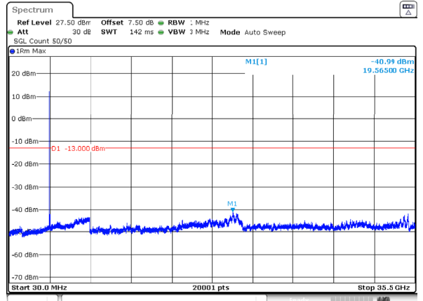
n77_1_60MHz_30kHz_3520MHz_DFT-s-OFDM QPSK_RB1@0 -40.99dBm
