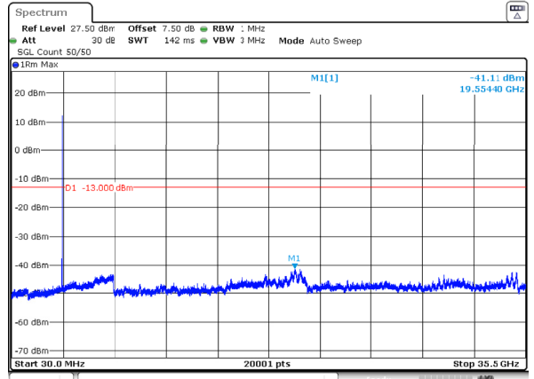
n77_1_20MHz_30kHz_3460MHz_DFT-s-OFDM QPSK_RB1@50 -41.11dBm
