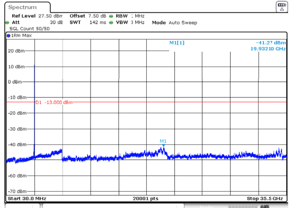
n77_1_60MHz_30kHz_3500MHz_DFT-s-OFDM QPSK_RB1@161 -41.27dBm
