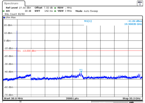
n77_1_70MHz_30kHz_3500MHz_DFT-s-OFDM QPSK_RB1@0 -41.05dBm
