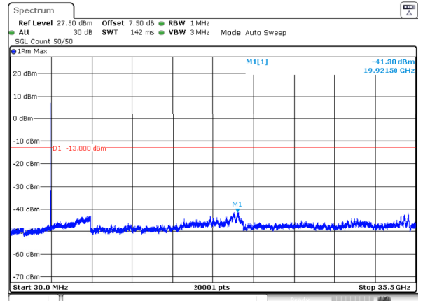
n77_1_10MHz_30kHz_3500MHz_DFT-s-OFDM QPSK_RB24@0 -41.30dBm
