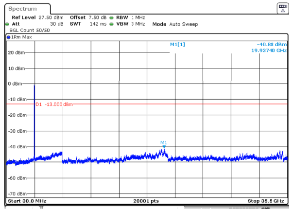
n77_1_60MHz_30kHz_3500MHz_DFT-s-OFDM QPSK_RB162@0 -40.88dBm
