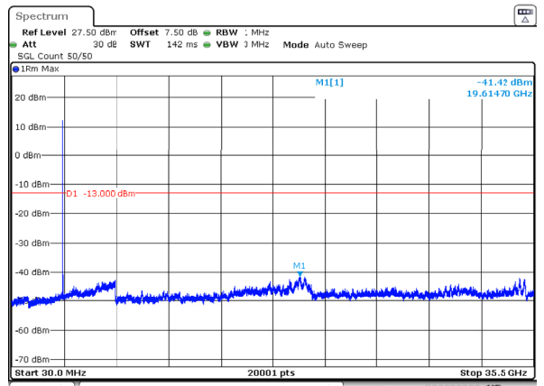
n77_1_30MHz_30kHz_3465MHz_DFT-s-OFDM QPSK_RB1@0 -41.42dBm
