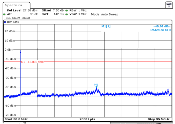
n77_1_70MHz_30kHz_3485MHz_DFT-s-OFDM QPSK_RB180@0 -40.99dBm
