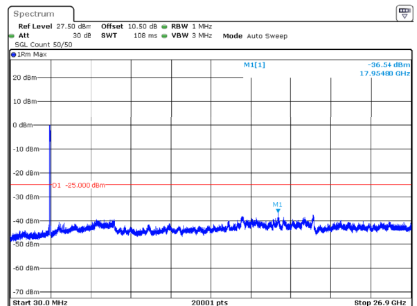
n41_80MHz_30kHz_2649.99MHz_DFT-s-OFDM QPSK_RB216@0 -36.54dBm
