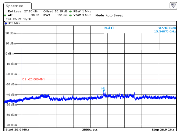
n41_20MHz_30kHz_2592.99MHz_DFT-s-OFDM QPSK_RB50@0 -37.45dBm
