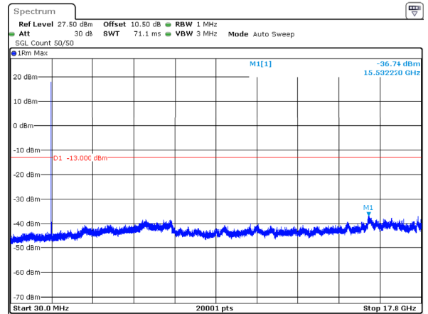
n66_25MHz_15kHz_1767.5MHz_DFT-s-OFDM QPSK_RB1@0 -36.74dBm
