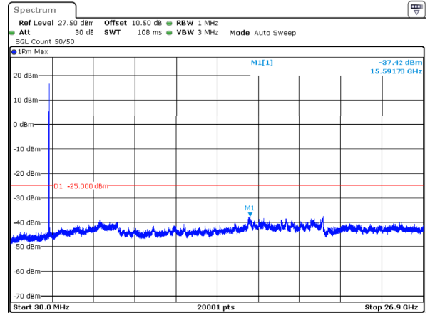
n41_40MHz_30kHz_2516.01MHz_DFT-s-OFDM QPSK_RB1@0 -37.42dBm
