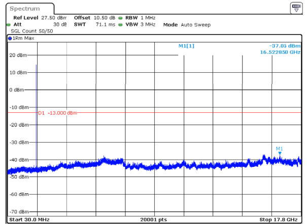
n66_5MHz_15kHz_1745MHz_DFT-s-OFDM QPSK_RB1@0 -37.05dBm
