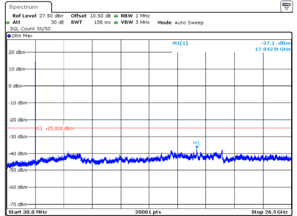
n41_20MHz_30kHz_2679.99MHz_DFT-s-OFDM QPSK_RB1@50 -37.11dBm
