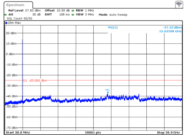
n41_40MHz_30kHz_2670MHz_DFT-s-OFDM QPSK_RB1@0 -37.52dBm
