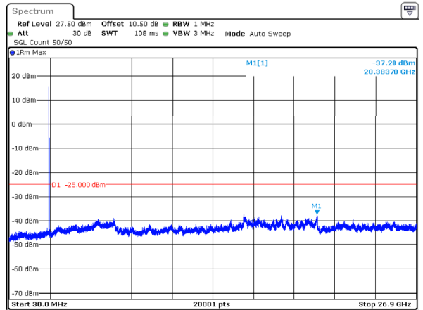
n41_60MHz_30kHz_2659.98MHz_DFT-s-OFDM QPSK_RB1@0 -37.28dBm
