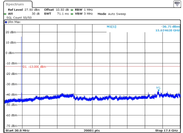
n66_25MHz_15kHz_1722.5MHz_DFT-s-OFDM QPSK_RB1@0 -36.75dBm
