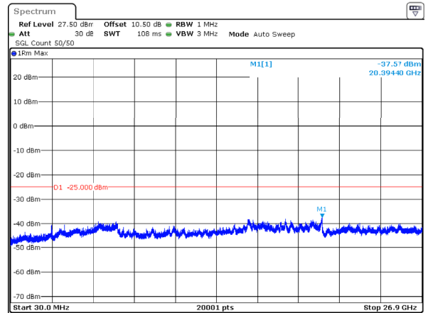
n41_80MHz_30kHz_2649.99MHz_DFT-s-OFDM QPSK_RB1@0 -37.57dBm
