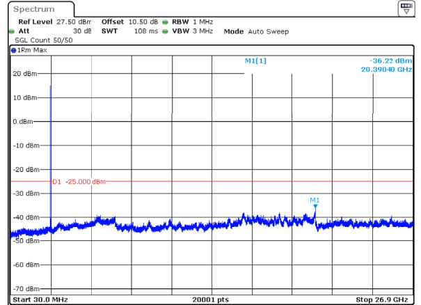
n41_30MHz_30kHz_2674.98MHz_DFT-s-OFDM QPSK_RB1@0 -36.22dBm
