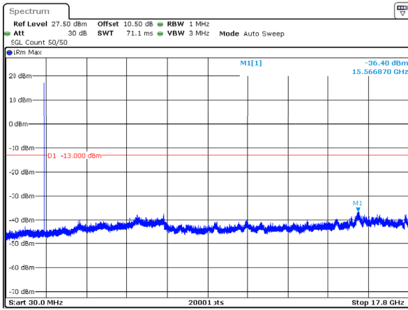
n66_5MHz_15kHz_1712.5MHz_DFT-s-OFDM QPSK_RB1@0 -36.40dBm
