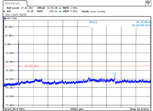
n41_50MHz_30kHz_2664.99MHz_DFT-s-OFDM QPSK_RB128@0 -36.73dBm
