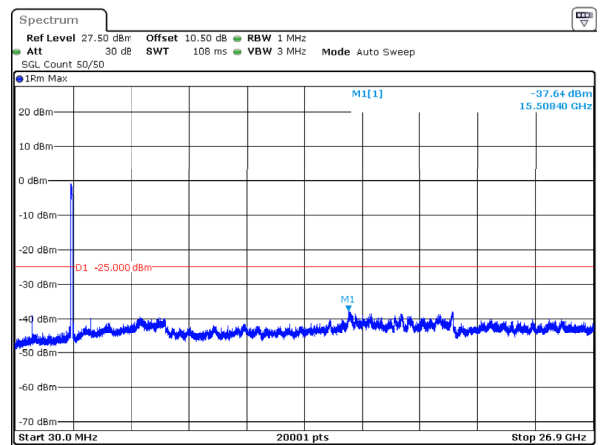
n41_100MHz_30kHz_2640MHz_DFT-s-OFDM QPSK_RB270@0 -37.64dBm
