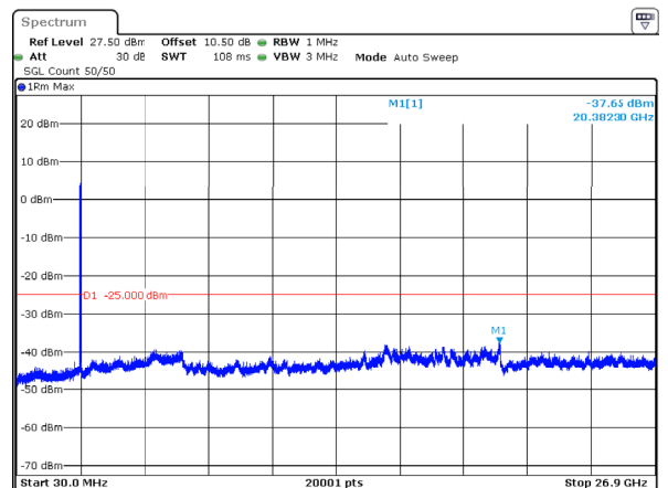
n41_30MHz_30kHz_2674.98MHz_DFT-s-OFDM QPSK_RB75@0 -37.65dBm
