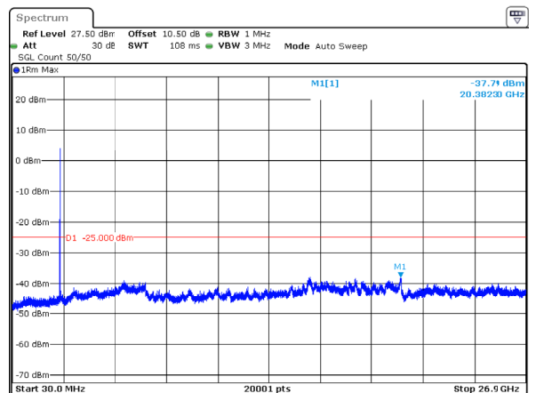
n41_30MHz_30kHz_2511MHz_DFT-s-OFDM QPSK_RB75@0 -37.79dBm
