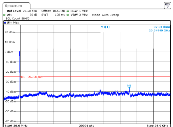
n41_80MHz_30kHz_2536.02MHz_DFT-s-OFDM QPSK_RB216@0 -37.30dBm
