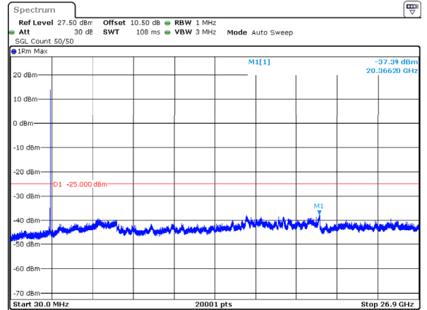
n41_30MHz_30kHz_2592.99MHz_DFT-s-OFDM QPSK_RB1@77 -37.39dBm
