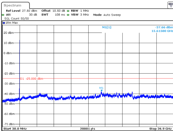
n41_40MHz_30kHz_2670MHz_DFT-s-OFDM QPSK_RB1@105 -37.66dBm
