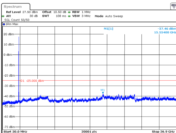
n41_50MHz_30kHz_2521.02MHz_DFT-s-OFDM QPSK_RB1@0 -37.46dBm
