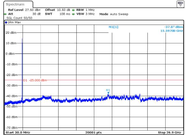
n41_80MHz_30kHz_2592.99MHz_DFT-s-OFDM QPSK_RB1@216 -37.87dBm
