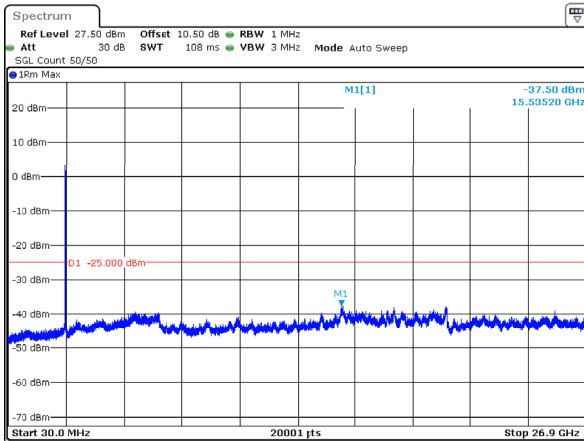
n41_40MHz_30kHz_2670MHz_DFT-s-OFDM QPSK_RB100@0 -37.50dBm
