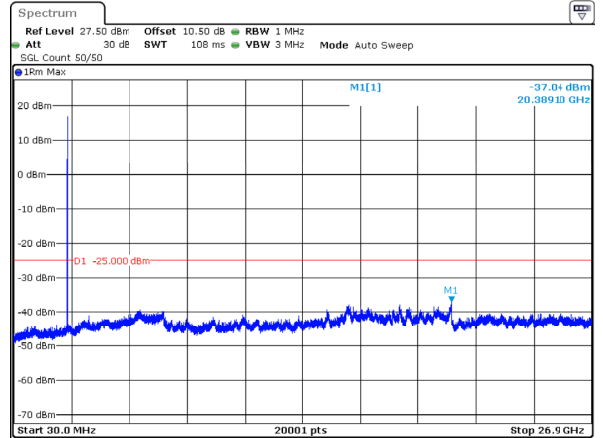
n41_30MHz_30kHz_2511MHz_DFT-s-OFDM QPSK_RB1@0 -37.04dBm
