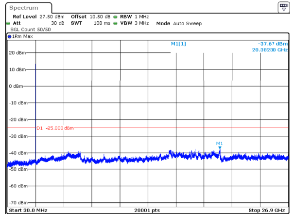
n41_15MHz_30kHz_2682.48MHz_DFT-s-OFDM QPSK_RB1@0 -37.67dBm
