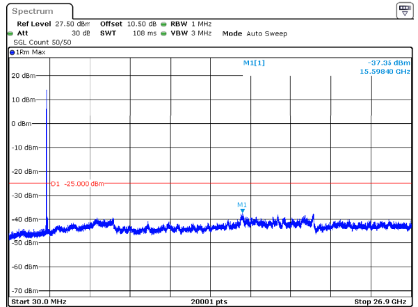
n41_80MHz_30kHz_2536.02MHz_DFT-s-OFDM QPSK_RB1@0 -37.35dBm
