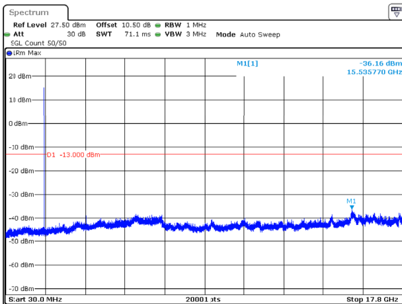
n66_5MHz_15kHz_1745MHz_DFT-s-OFDM QPSK_RB1@24 -36.16dBm
