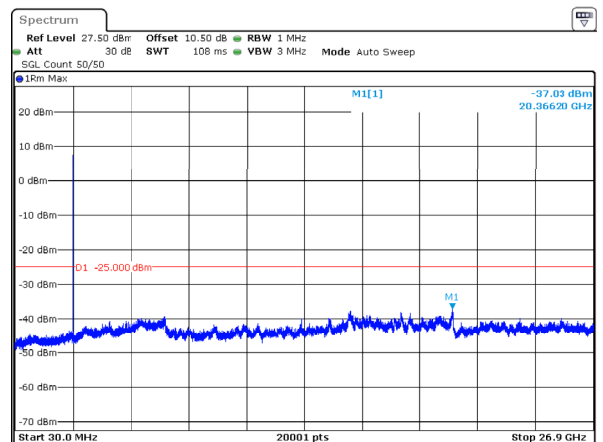
n41_15MHz_30kHz_2682.48MHz_DFT-s-OFDM QPSK_RB36@0 -37.03dBm
