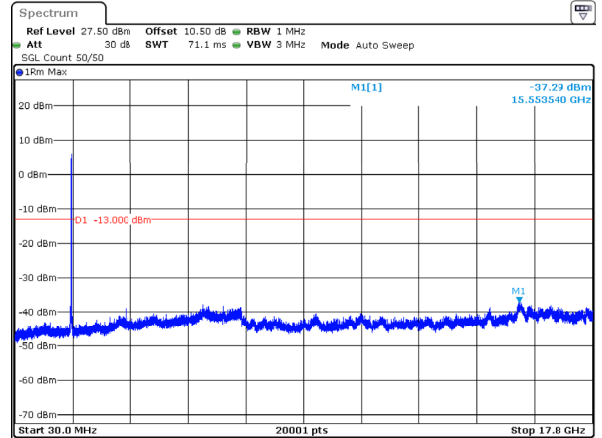
n66_25MHz_15kHz_1745MHz_DFT-s-OFDM QPSK_RB128@0 -37.29dBm
