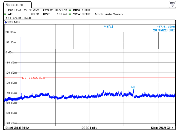
n41_100MHz_30kHz_2640MHz_DFT-s-OFDM QPSK_RB1@0 -37.41dBm
