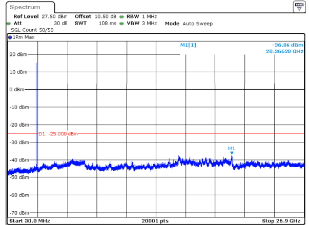
n41_50MHz_30kHz_2592.99MHz_DFT-s-OFDM QPSK_RB1@0 -36.86dBm
