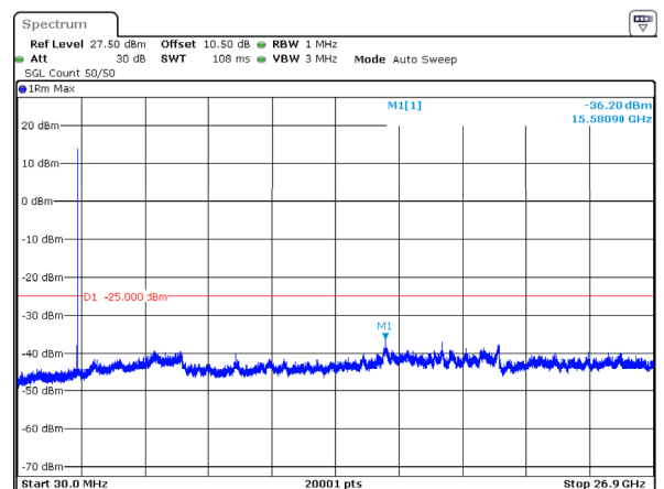
n41_50MHz_30kHz_2521.02MHz_DFT-s-OFDM QPSK_RB1@132 -36.20dBm
