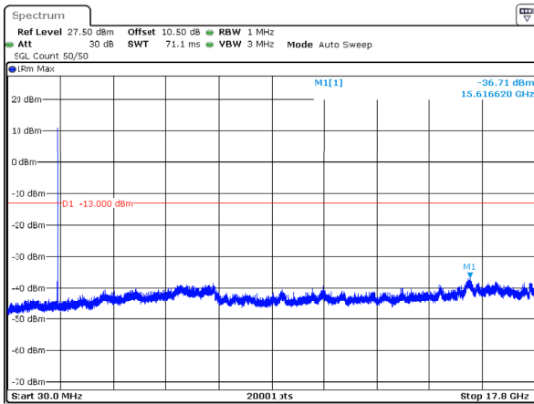
n66_5MHz_15kHz_1712.5MHz_DFT-s-OFDM QPSK_RB25@0 -36.71dBm
