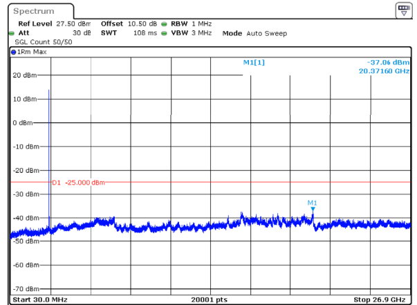
n41_20MHz_30kHz_2592.99MHz_DFT-s-OFDM QPSK_RB1@0 -37.06dBm
