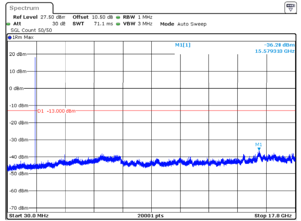
n66_5MHz_15kHz_1712.5MHz_DFT-s-OFDM QPSK_RB1@24 -36.28dBm
