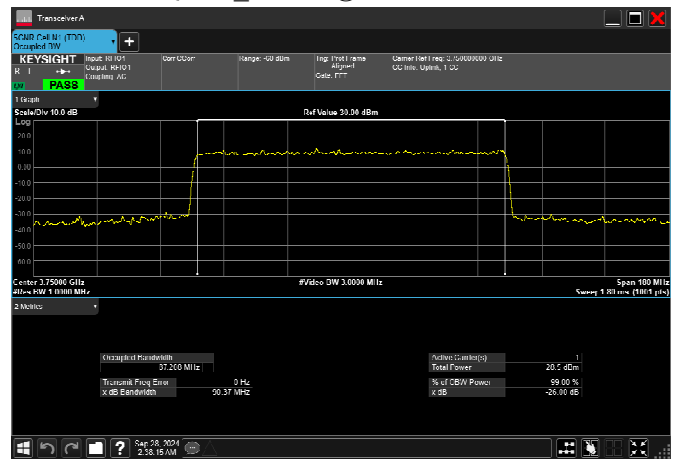
n78_3_90MHz_30kHz_3750MHz_CP-OFDM QPSK_RB245@0 87.208MHz
