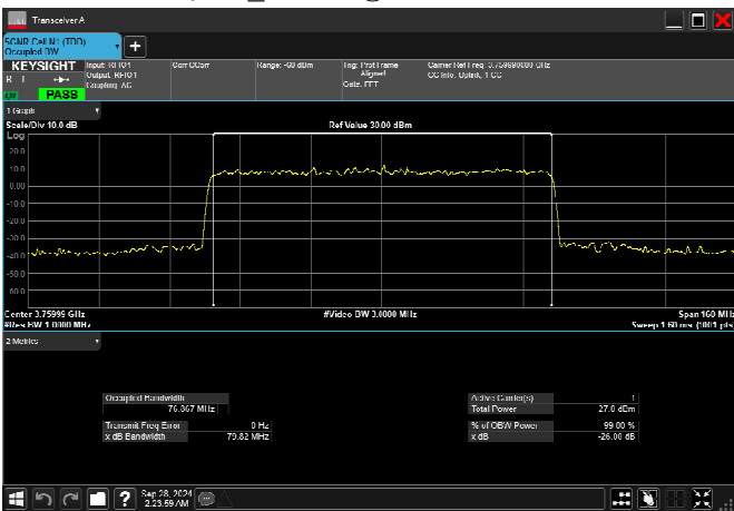
n78_3_80MHz_30kHz_3760MHz_DFT-s-OFDM 256 QAM_RB216@0 76.867MHz
