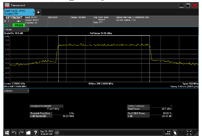
n78_3_80MHz_30kHz_3760MHz_CP-OFDM QPSK_RB217@0 77.447MHz
