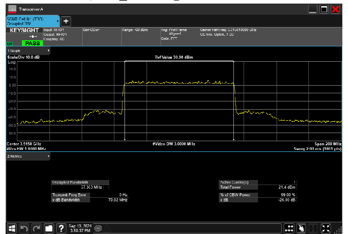
n78_1_70MHz_30kHz_3515MHz_CP-OFDM QPSK_RB189@0 67.363MHz
