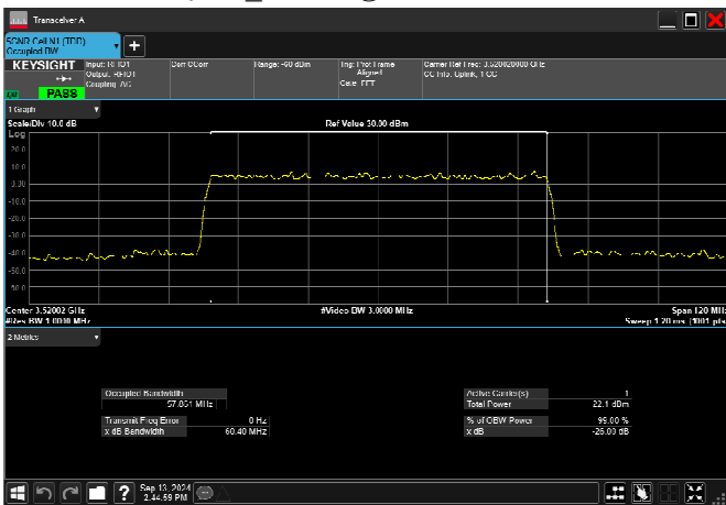
n78_1_60MHz_30kHz_3520MHz_CP-OFDM 64 QAM_RB162@0 57.861MHz
