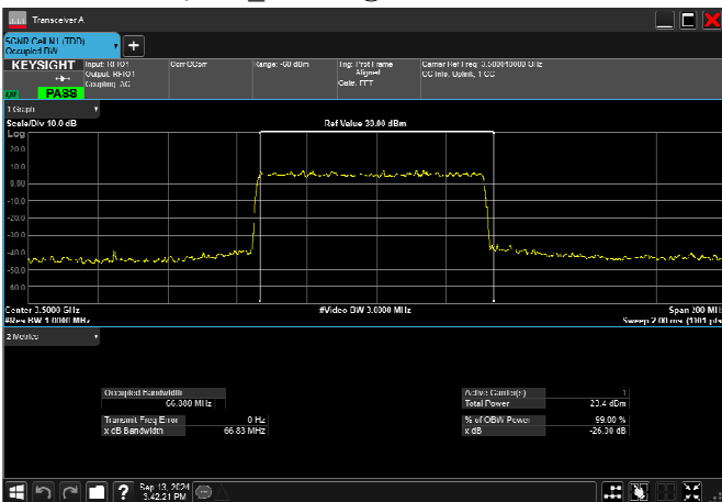
n78_1_70MHz_30kHz_3500MHz_DFT-s-OFDM QPSK_RB180@0 66.880MHz
