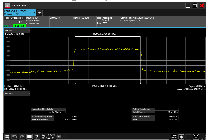
n78_1_70MHz_30kHz_3485MHz_CP-OFDM QPSK_RB189@0 67.327MHz
