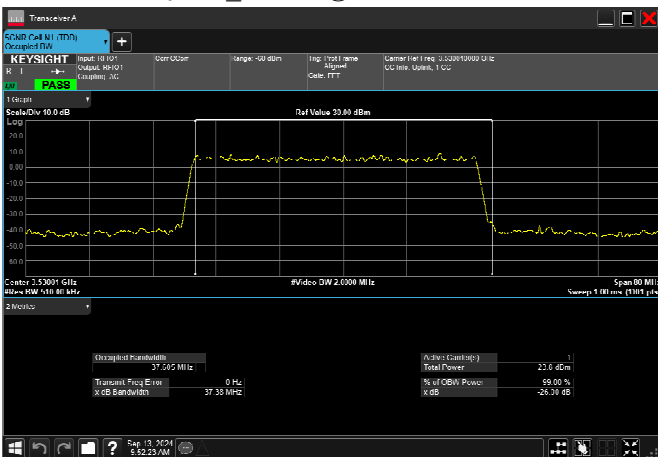
n78_1_40MHz_30kHz_3530MHz_DFT-s-OFDM QPSK_RB100@0 37.605MHz
