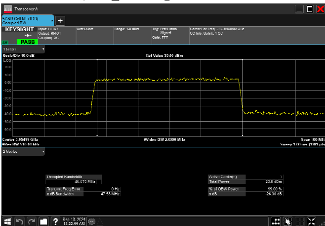
n77_3_50MHz_30kHz_3955MHz_DFT-s-OFDM QPSK_RB128@0 46.675MHz
