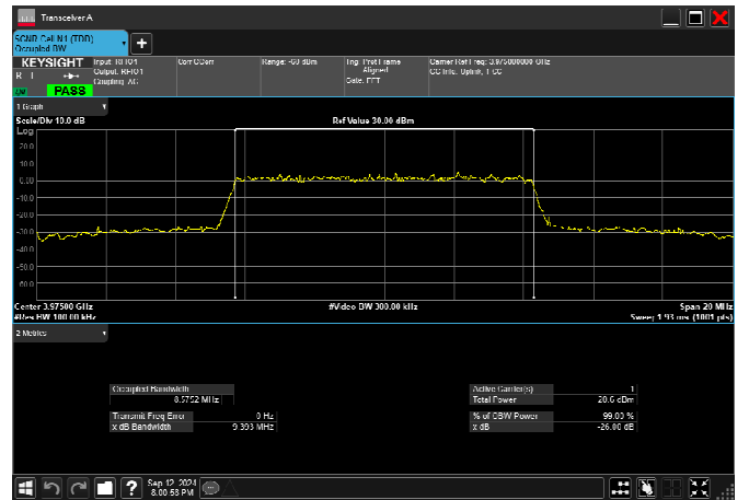
n77_3_10MHz_30kHz_3975MHz_CP-OFDM QPSK_RB24@0 8.575MHz
