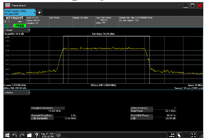
n77_3_15MHz_30kHz_3707.5MHz_DFT-s-OFDM 16 QAM_RB36@0 13.500MHz
