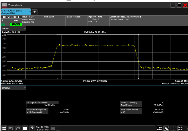
n77_3_15MHz_30kHz_3707.5MHz_DFT-s-OFDM QPSK_RB36@0 13.451MHz
