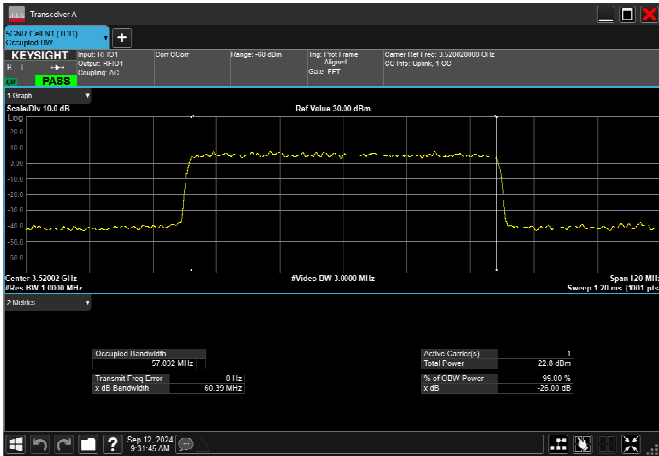
n77_1_60MHz_30kHz_3520MHz_CP-OFDM QPSK_RB162@0 57.602MHz
