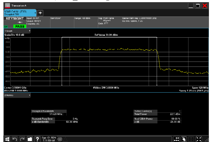
n77_1_60MHz_30kHz_3500MHz_CP-OFDM QPSK_RB162@0 57.628MHz
