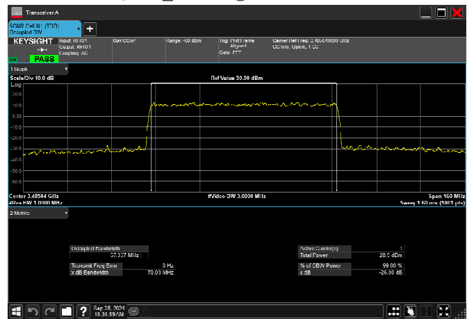
n77_1_70MHz_30kHz_3485MHz_CP-OFDM QPSK_RB189@0 67.337MHz
