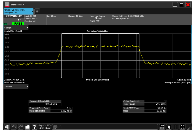
n77_1_10MHz_30kHz_3455MHz_CP-OFDM 256 QAM_RB24@0 8.608MHz
