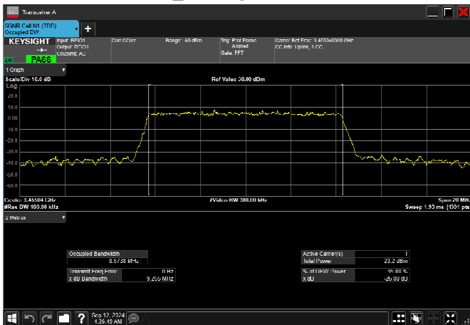
n77_1_10MHz_30kHz_3455MHz_DFT-s-OFDM QPSK_RB24@0 8.574MHz
