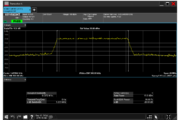
n77_1_10MHz_30kHz_3455MHz_CP-OFDM 16 QAM_RB24@0 8.565MHz
