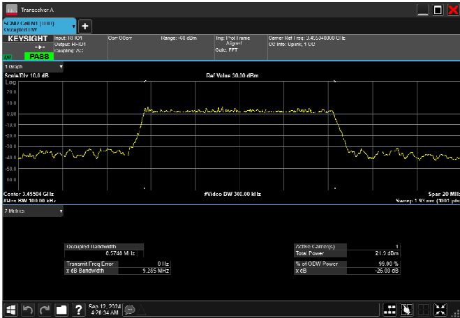
n77_1_10MHz_30kHz_3455MHz_CP-OFDM QPSK_RB24@0 8.536MHz
