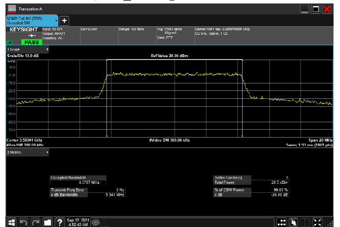
n77_1_10MHz_30kHz_3500MHz_CP-OFDM QPSK_RB24@0 8.579MHz
