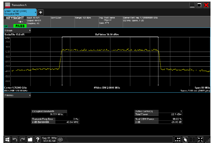
n66_40MHz_15kHz_1760MHz_CP-OFDM QPSK_RB216@0 38.561MHz
