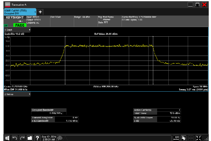
n66_5MHz_15kHz_1712.5MHz_CP-OFDM QPSK_RB25@0 4.466MHz
