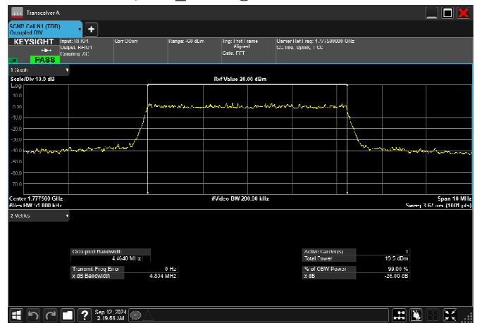
n66_5MHz_15kHz_1777.5MHz_CP-OFDM QPSK_RB25@0 4.464MHz
