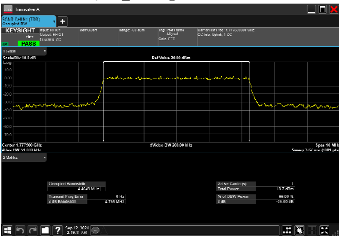
n66_5MHz_15kHz_1777.5MHz_DFT-s-OFDM 256 QAM_RB25@0 4.465MHz
