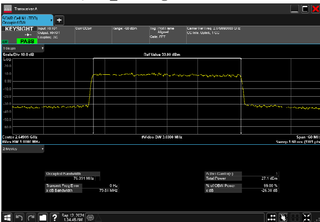
n41_80MHz_30kHz_2649.99MHz_DFT-s-OFDM QPSK_RB216@0 76.891MHz
