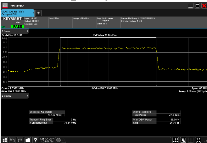
n41_80MHz_30kHz_2536.02MHz_DFT-s-OFDM QPSK_RB216@0 77.140MHz
