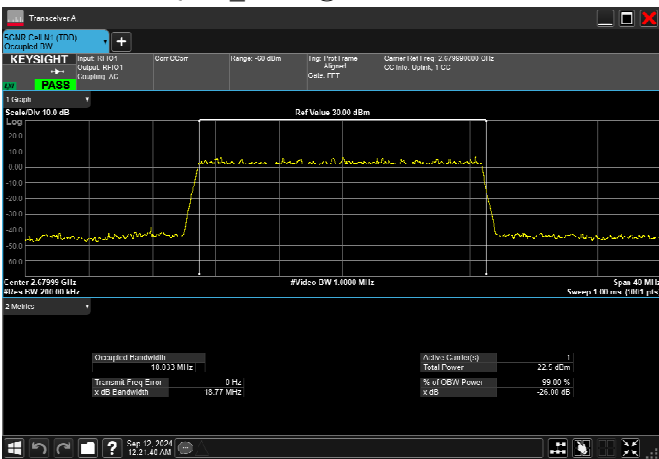
n41_20MHz_30kHz_2679.99MHz_DFT-s-OFDM 256 QAM_RB50@0 18.033MHz
