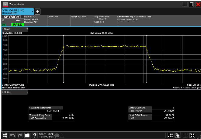
n41_10MHz_30kHz_2685MHz_DFT-s-OFDM 16 QAM_RB24@0 8.576MHz
