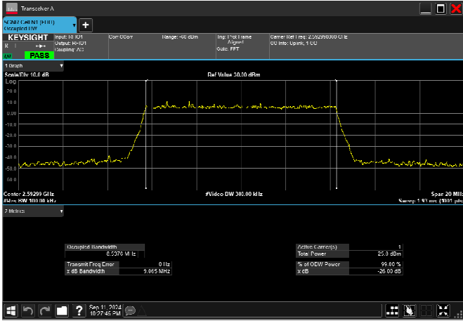
n41_10MHz_30kHz_2592.99MHz_CP-OFDM QPSK_RB24@0 8.603MHz
