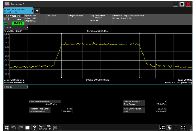
n41_10MHz_30kHz_2685MHz_DFT-s-OFDM 64 QAM_RB24@0 8.580MHz
