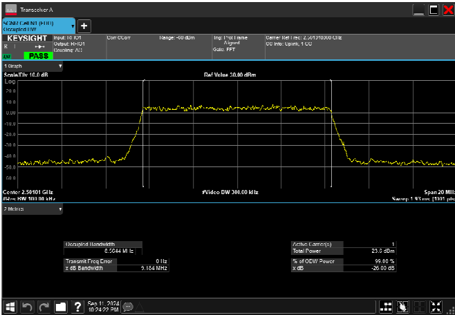
n41_10MHz_30kHz_2501.01MHz_CP-OFDM 256 QAM_RB24@0 8.610MHz
