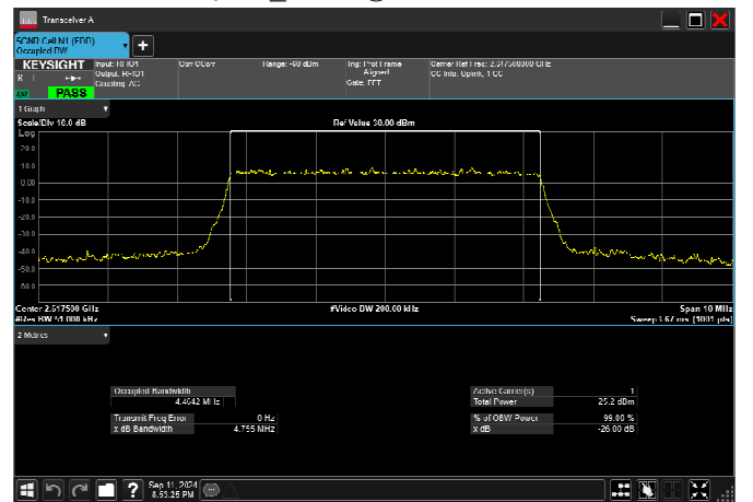
n38_5MHz_15kHz_2617.5MHz_DFT-s-OFDM 16 QAM_RB25@0 4.464MHz
