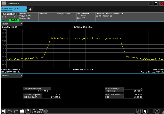
n38_5MHz_15kHz_2617.5MHz_CP-OFDM QPSK_RB25@0 4.482MHz
