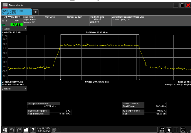
n38_10MHz_30kHz_2595MHz_DFT-s-OFDM QPSK_RB24@0 8.573MHz
