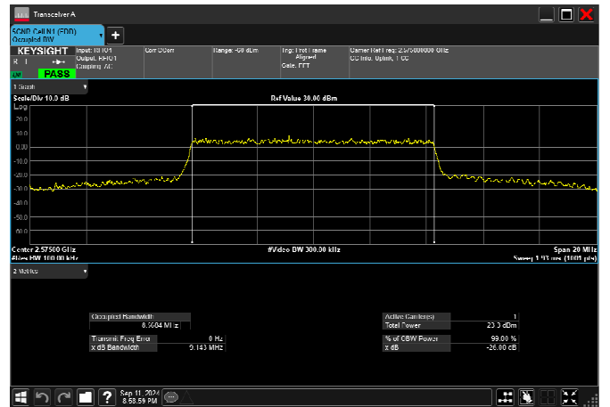
n38_10MHz_30kHz_2575MHz_CP-OFDM QPSK_RB24@0 8.568MHz
