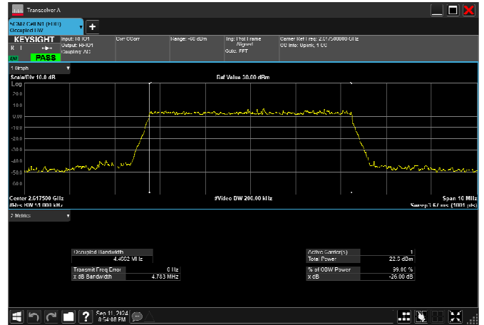
n38_5MHz_15kHz_2617.5MHz_CP-OFDM 16 QAM_RB25@0 4.465MHz
