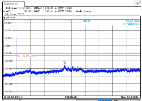
1_5MHz_Middle_QPSK_25@0
