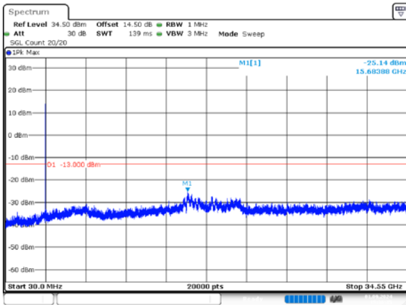
1_10MHz_Low_QPSK_1@0
