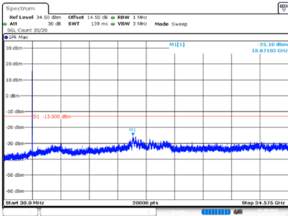
1_15MHz_Low_QPSK_1@0
