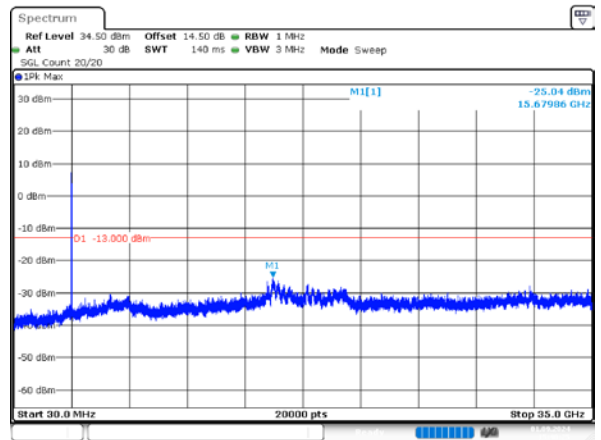
1_15MHz_Middle_QPSK_75@0
