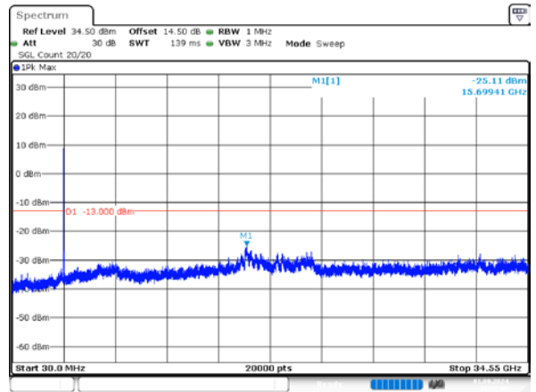
1_10MHz_Low_QPSK_50@0
