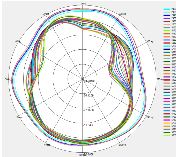
BT&WIFI-2.4G & 5G Phi=90deg
