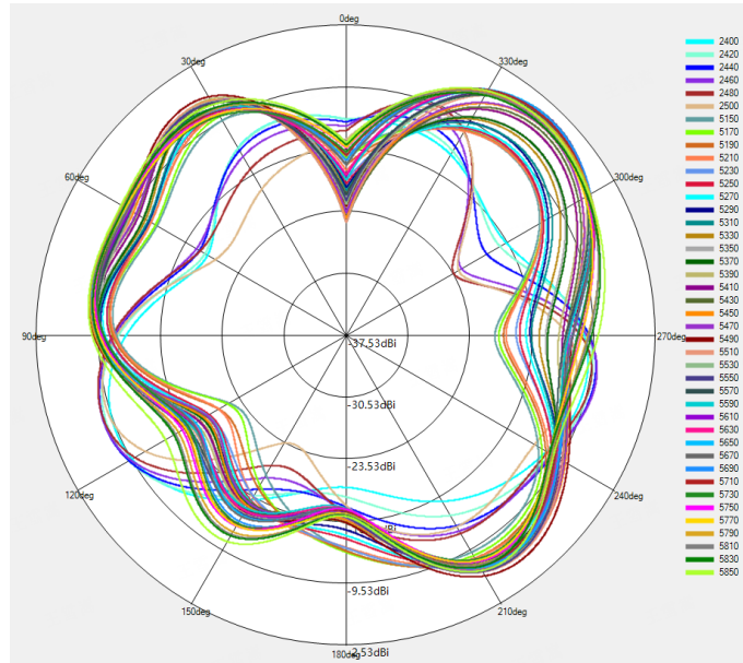
BT&WIFI-2.4G & 5G Theta=90deg
