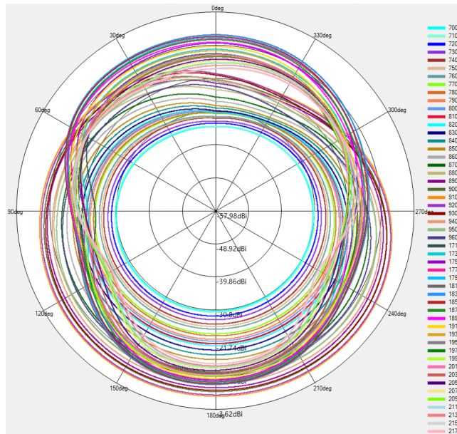
900R/PCS1900/WCDMA B2/LTE B2 Theta=90deg
