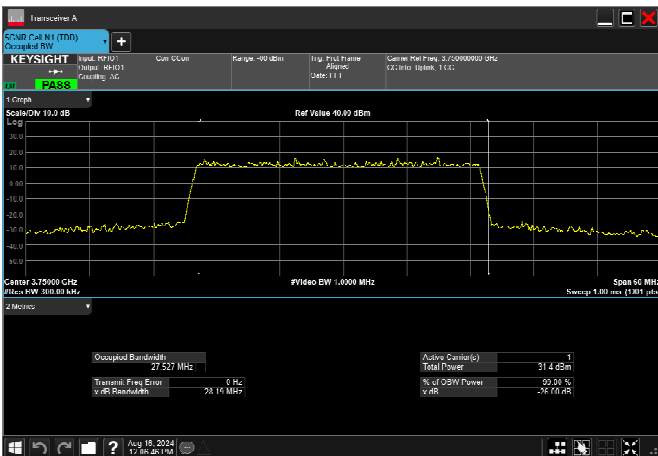
n78_3_30MHz_30kHz_3750MHz_DFT-s-OFDM QPSK_RB75@0 27.527MHz
