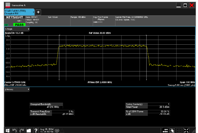
n78_3_50MHz_30kHz_3750MHz_CP-OFDM 256 QAM_RB133@0 47.290MHz
