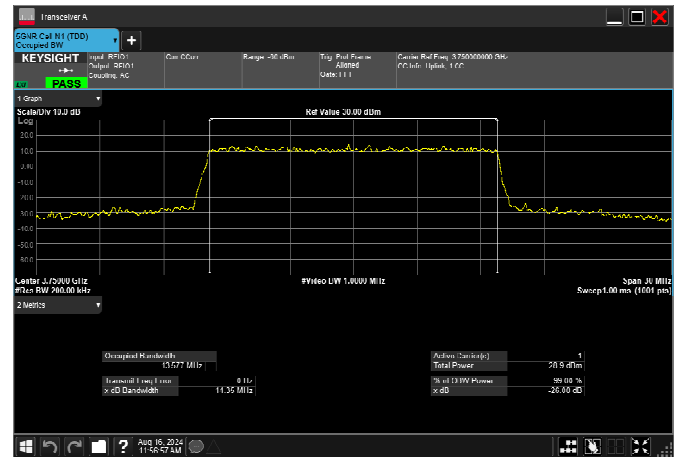
n78_3_15MHz_30kHz_3750MHz_CP-OFDM 256 QAM_RB38@0 13.527MHz
