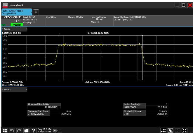
n78_3_20MHz_30kHz_3750MHz_DFT-s-OFDM 256 QAM_RB50@0 18.006MHz
