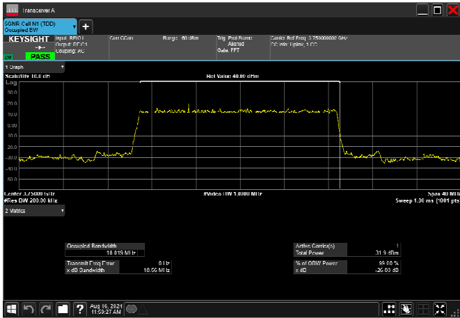
n78_3_20MHz_30kHz_3750MHz_DFT-s-OFDM 16 QAM_RB50@0 18.094MHz
