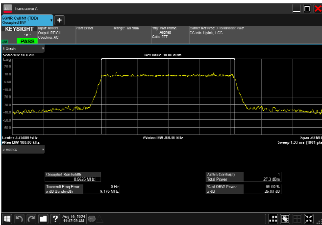
n78_3_10MHz_30kHz_3750MHz_DFT-s-OFDM 256 QAM_RB24@0 8.563MHz
