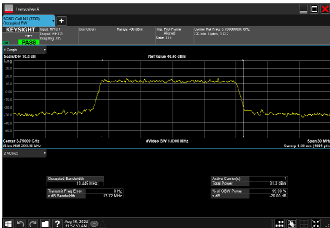
n78_3_15MHz_30kHz_3750MHz_DFT-s-OFDM QPSK_RB36@0 13.445MHz
