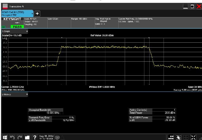
n78_3_15MHz_30kHz_3750MHz_CP-OFDM 64 QAM_RB38@0 13.585MHz
