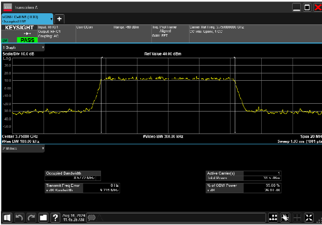
n78_3_10MHz_30kHz_3750MHz_DFT-s-OFDM 16 QAM_RB24@0 8.566MHz
