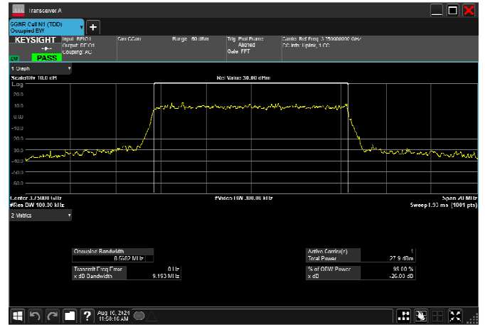
n78_3_15MHz_30kHz_3750MHz_DFT-s-OFDM \pi/2 BPSK_RB36@0 13.460MHz
