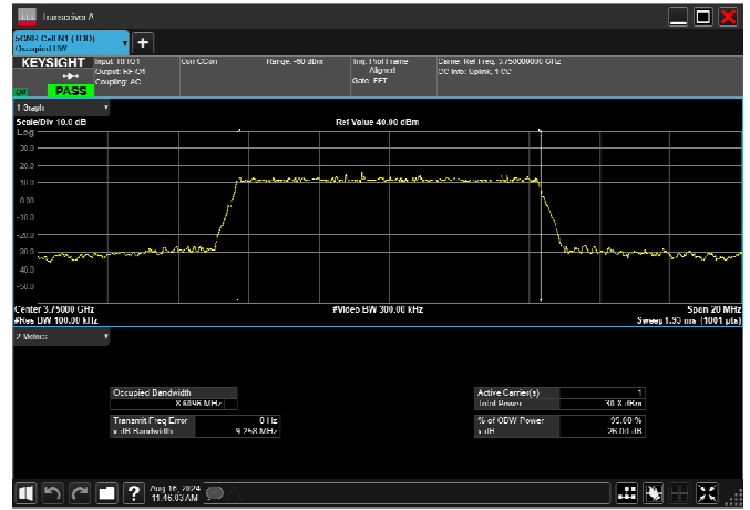
n78_3_10MHz_30kHz_3750MHz_DFT-s-OFDM 64 QAM_RB24@0 8.560MHz
