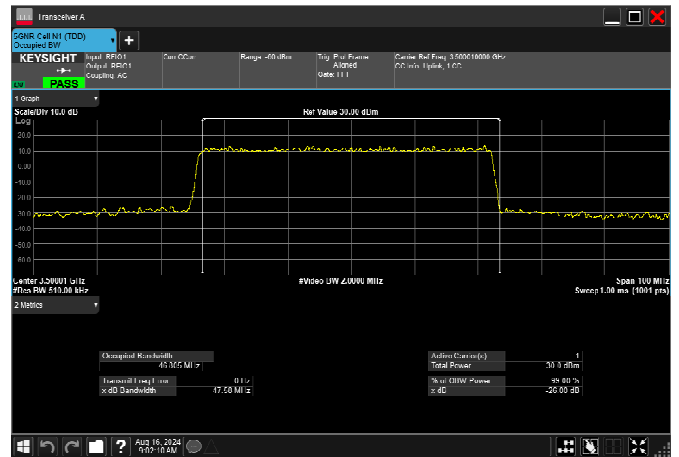
n78_1_50MHz_30kHz_3500MHz_CP-OFDM QPSK_RB133@0 47.289MHz
