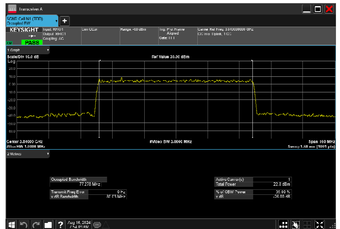
n77_3_80MHz_30kHz_3840MHz_CP-OFDM QPSK_RB217@0 77.278MHz
