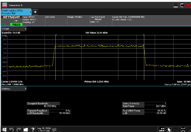
n77_3_90MHz_30kHz_3840MHz_DFT-s-OFDM QPSK_RB243@0 86.783MHz
