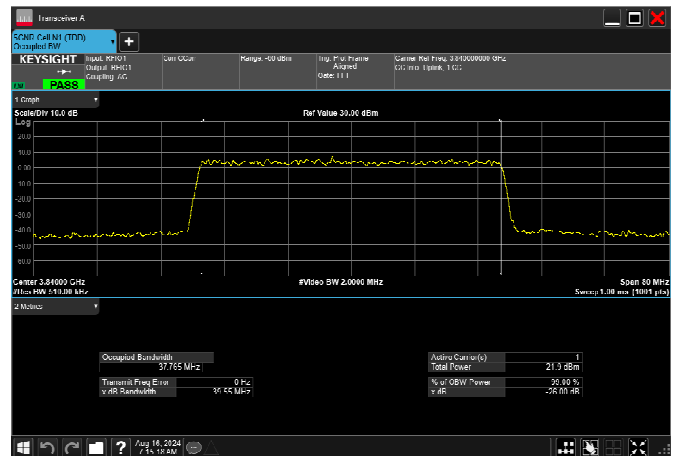
n77_3_40MHz_30kHz_3840MHz_CP-OFDM QPSK_RB106@0 37.765MHz
