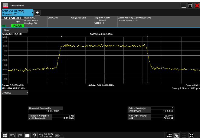
n77_3_20MHz_30kHz_3840MHz_DFT-s-OFDM 256 QAM_RB50@0 18.007MHz
