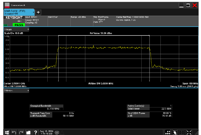
n77_1_90MHz_30kHz_3500MHz_CP-OFDM QPSK_RB245@0 87.190MHz
