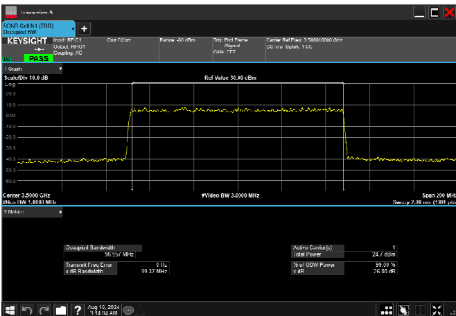
n77_1_100MHz_30kHz_3500MHz_DFT-s-OFDM QPSK_RB270@0 96.557MHz
