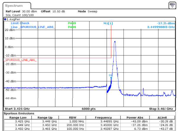
n78_1_15MHz_30kHz_3457.5MHz_DFT-s-OFDM QPSK_RB1@0 -37.255MHz
