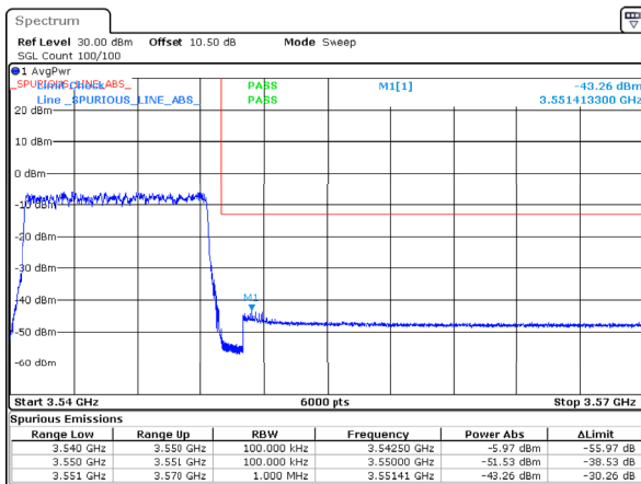
n78_1_10MHz_30kHz_3455MHz_DFT-s-OFDM QPSK_RB24@0 -43.256MHz
