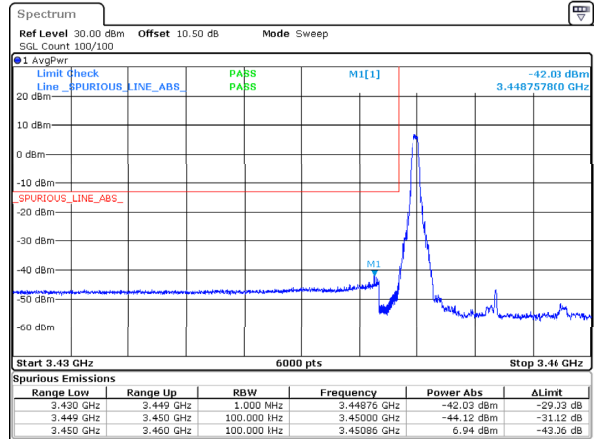
n78_1_10MHz_30kHz_3455MHz_DFT-s-OFDM QPSK_RB1@0 -42.035MHz
