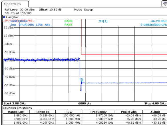
n77_3_100MHz_30kHz_3930MHz_DFT-s-OFDM QPSK_RB270@0 -46.202MHz
