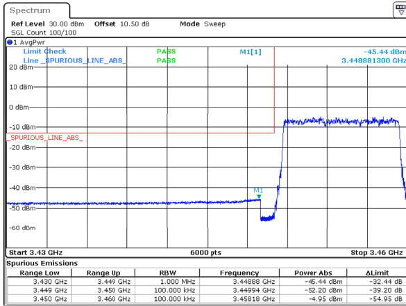
n78_1_10MHz_30kHz_3455MHz_DFT-s-OFDM QPSK_RB24@0 -45.439MHz
