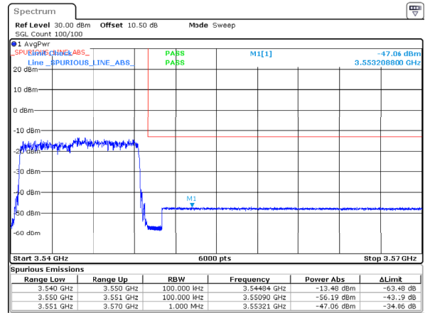
n77_1_10MHz_30kHz_3545MHz_DFT-s-OFDM QPSK_RB24@0 -47.063MHz
