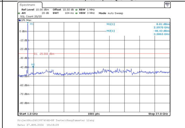
1000.0MHz-27000.0MHz Band 38 20MHz/2585.1/Mid QPSK 100@0 Band 38 20MHz/2604.9/Mid QPSK 100@0
