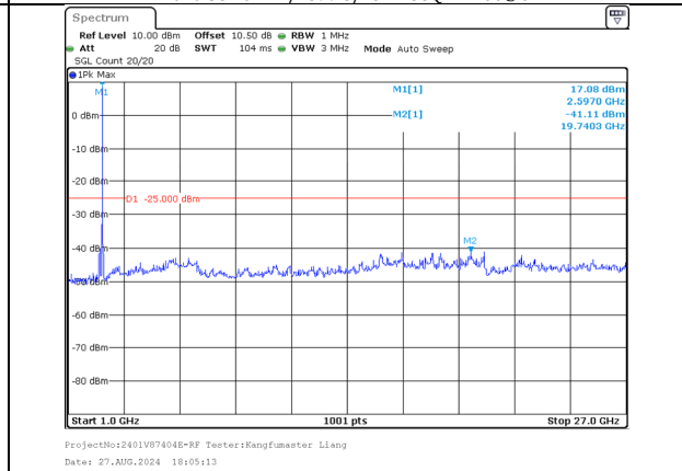
1000.0MHz-27000.0MHz Band 38 15MHz/2587.5/Mid QPSK 1@74 Band 38 15MHz/2602.5/Mid QPSK 1@0
