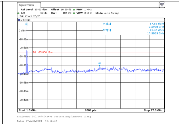
1000.0MHz-27000.0MHz Band 38 20MHz/2585.1/Mid QPSK 1@99 Band 38 20MHz/2604.9/Mid QPSK 1@0
