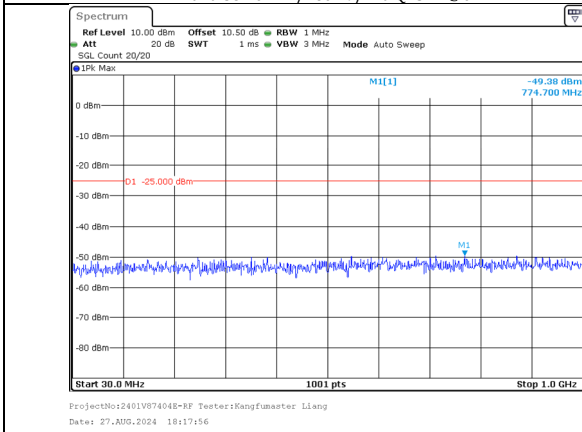
30.0MHz-1000.0MHz Band 38 20MHz/2585.1/Mid QPSK 100@0 Band 38 20MHz/2604.9/Mid QPSK 100@0
