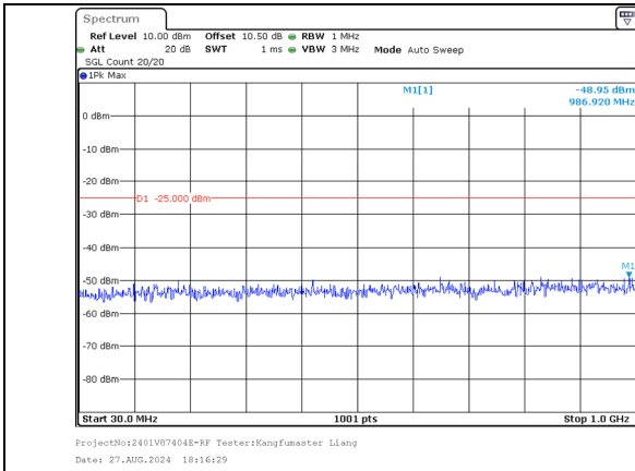
30.0MHz-1000.0MHz Band 38 20MHz/2585.1/Mid QPSK 1@99 Band 38 20MHz/2604.9/Mid QPSK 1@0
