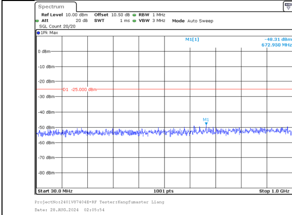
30.0MHz-1000.0MHz Band 7 20MHz/2525.1/Mid QPSK 1@99 Band 7 20MHz/2544.9/Mid QPSK 1@0
