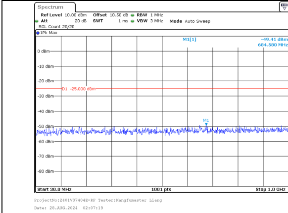
30.0MHz-1000.0MHz Band 7 20MHz/2525.1/Mid QPSK 100@0 Band 7 20MHz/2544.9/Mid QPSK 100@0
