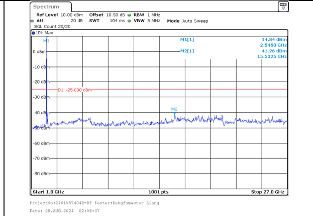
1000.0MHz-27000.0MHz Band 7 20MHz/2525.1/Mid QPSK 1@99 Band 7 20MHz/2544.9/Mid QPSK 1@0
