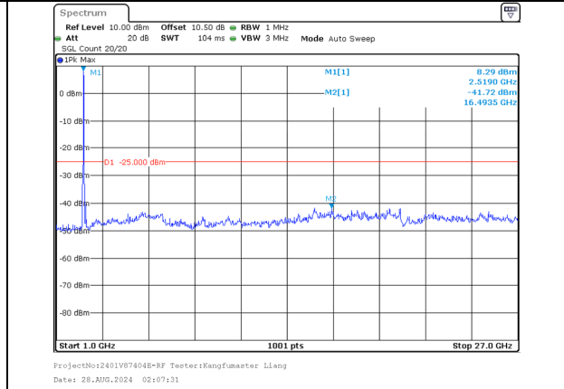
1000.0MHz-27000.0MHz Band 7 20MHz/2525.1/Mid QPSK 100@0 Band 7 20MHz/2544.9/Mid QPSK 100@0
