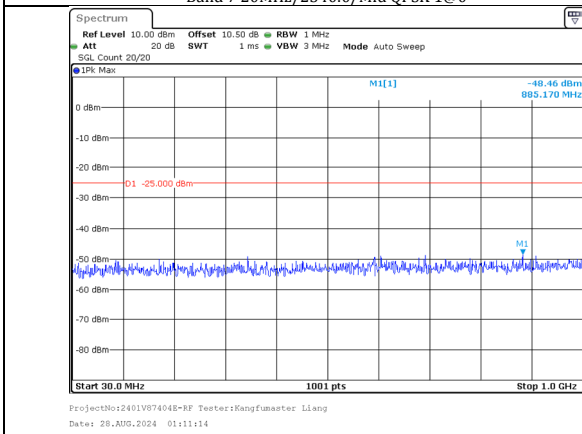
30.0MHz-1000.0MHz Band 7 10MHz/2525.6/Mid QPSK 50@0 Band 7 20MHz/2540.0/Mid QPSK 100@0
