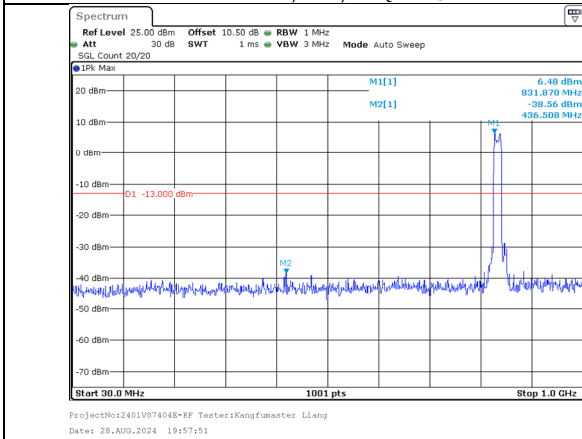
30.0MHz-1000.0MHz Band 5 10MHz/834.0/Mid QPSK 50@0 Band 5 5MHz/841.2/Mid QPSK 25@0
