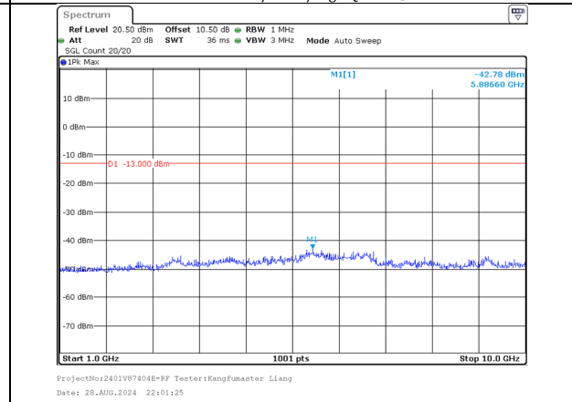
1000.0MHz-10000.0MHz Band 5 10MHz/834.1/High QPSK 50@0 Band 5 10MHz/844.0/High QPSK 50@0
