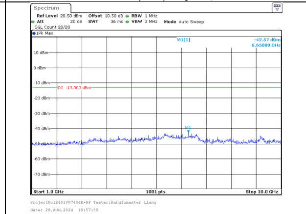
1000.0MHz-10000.0MHz Band 5 10MHz/834.0/Mid QPSK 50@0 Band 5 5MHz/841.2/Mid QPSK 25@0
