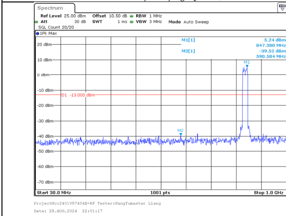
30.0MHz-1000.0MHz Band 5 10MHz/834.1/High QPSK 50@0 Band 5 10MHz/844.0/High QPSK 50@0
