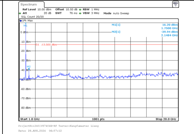
1000.0MHz-20000.0MHz Band 66 15MHz/1747.5/Mid QPSK 1@74 Band 66 15MHz/1762.5/Mid QPSK 1@0
