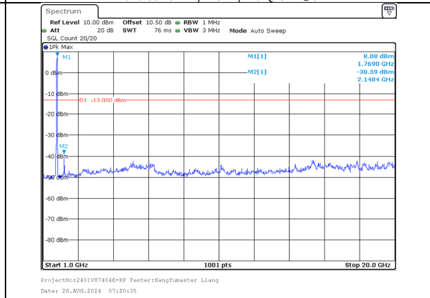
1000.0MHz-20000.0MHz Band 66 20MHz/1747.6/Mid QPSK 100@0 Band 66 15MHz/1764.7/Mid QPSK 100@0
