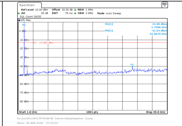
1000.0MHz-20000.0MHz Band 66 20MHz/1747.6/Mid QPSK 1@99 Band 66 15MHz/1764.7/Mid QPSK 1@0
