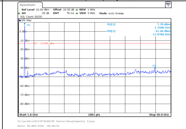
1000.0MHz-20000.0MHz Band 66 10MHz/1745.6/Mid QPSK 50@0 Band 66 20MHz/1760.0/Mid QPSK 100@0
