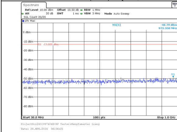
30.0MHz-1000.0MHz Band 66 10MHz/1745.6/Mid QPSK 50@0 Band 66 20MHz/1760.0/Mid QPSK 100@0
