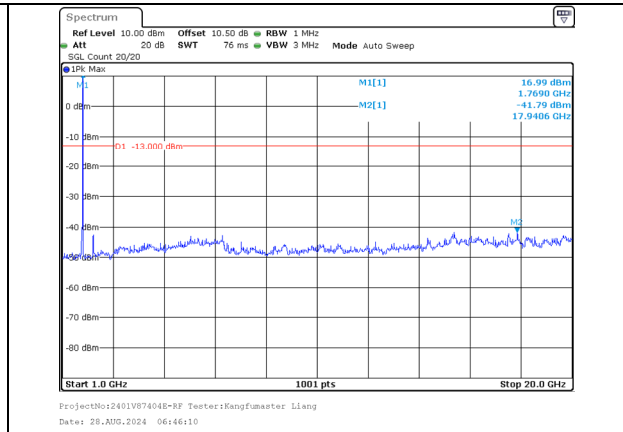
1000.0MHz-20000.0MHz Band 66 20MHz/1750.1/Mid QPSK 1@99 Band 66 10MHz/1764.5/Mid QPSK 1@0
