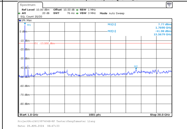
1000.0MHz-20000.0MHz Band 66 20MHz/1750.1/Mid QPSK 100@0 Band 66 10MHz/1764.5/Mid QPSK 100@0
