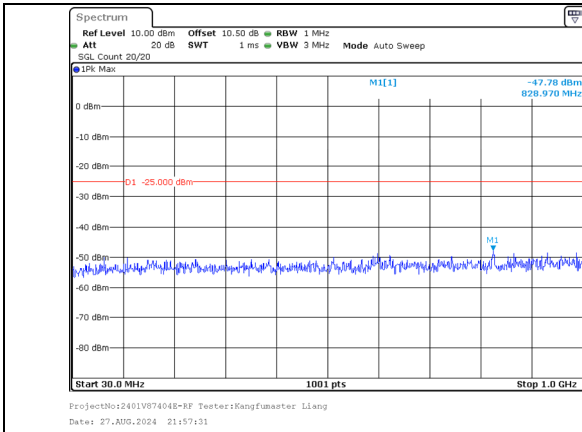
30.0MHz-1000.0MHz Band 41 20MHz/2583.1/Mid QPSK 1@99 Band 41 20MHz/2602.9/Mid QPSK 1@0
