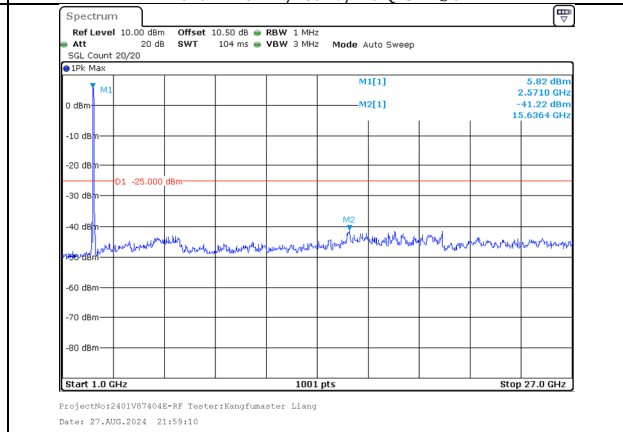
1000.0MHz-27000.0MHz Band 41 20MHz/2583.1/Mid QPSK 100@0 Band 41 20MHz/2602.9/Mid QPSK 100@0
