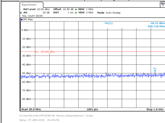
30.0MHz-1000.0MHz Band 41 20MHz/2583.1/Mid QPSK 100@0 Band 41 20MHz/2602.9/Mid QPSK 100@0
