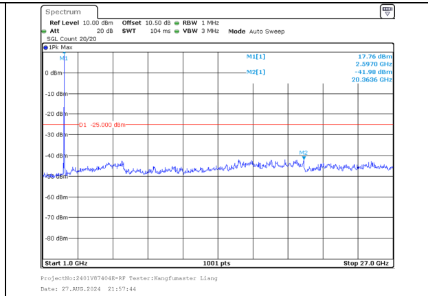
1000.0MHz-27000.0MHz Band 41 20MHz/2583.1/Mid QPSK 1@99 Band 41 20MHz/2602.9/Mid QPSK 1@0
