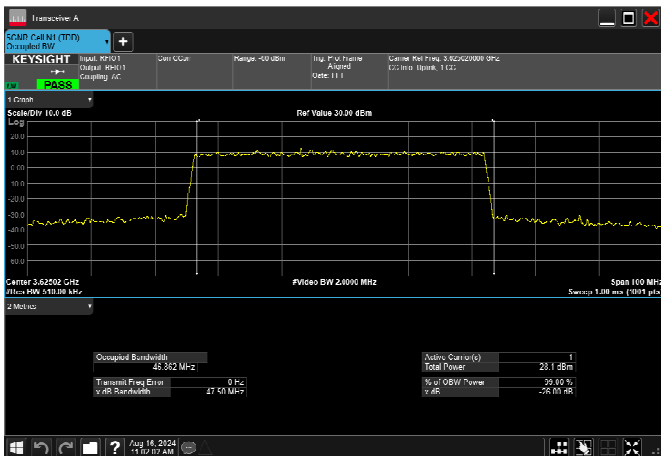
n78_2_50MHz_30kHz_3625MHz_DFT-s-OFDM 256 QAM_RB128@0 46.862MHz
