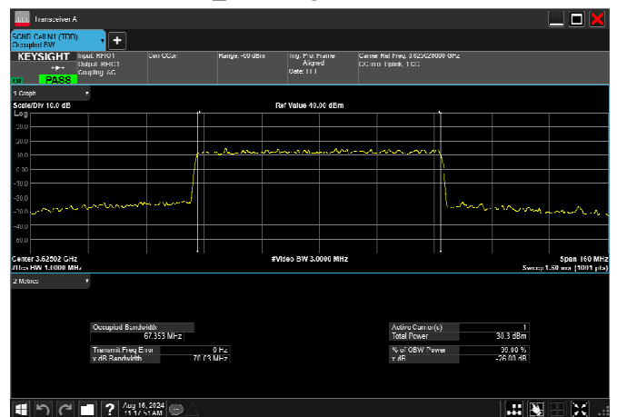
n78_2_70MHz_30kHz_3625MHz_CP-OFDM QPSK_RB189@0 67.353MHz
