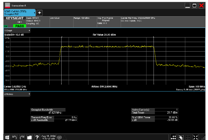
n78_2_50MHz_30kHz_3625MHz_CP-OFDM QPSK_RB133@0 47.429MHz
