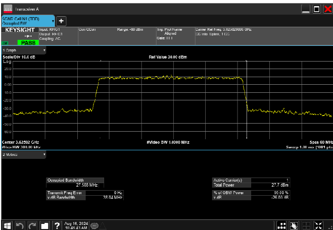
n78_2_30MHz_30kHz_3625MHz_DFT-s-OFDM 256 QAM_RB75@0 27.508MHz
