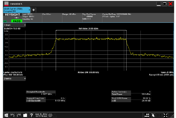
n78_2_10MHz_30kHz_3625MHz_CP-OFDM 256 QAM_RB24@0 8.609MHz
