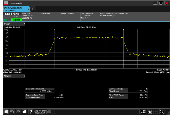
n78_2_10MHz_30kHz_3625MHz_CP-OFDM 16 QAM_RB24@0 8.568MHz
