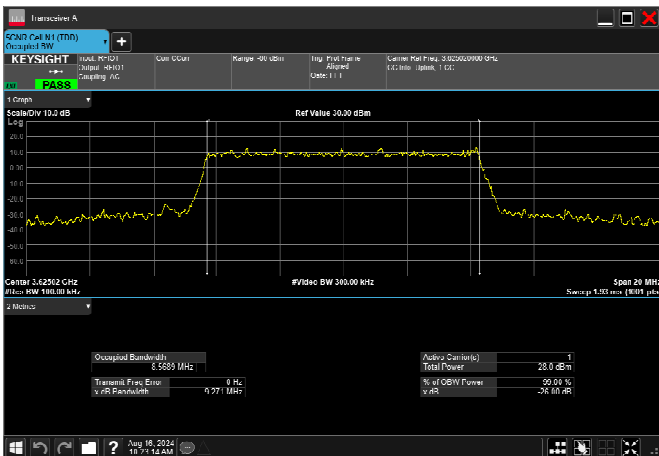
n78_2_10MHz_30kHz_3625MHz_CP-OFDM 64 QAM_RB24@0 8.569MHz
