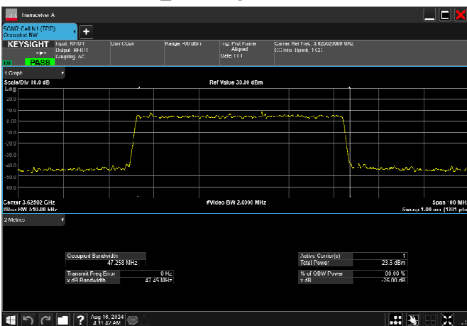
n77_2_50MHz_30kHz_3625MHz_DFT-s-OFDM QPSK_RB128@0 47.258MHz
