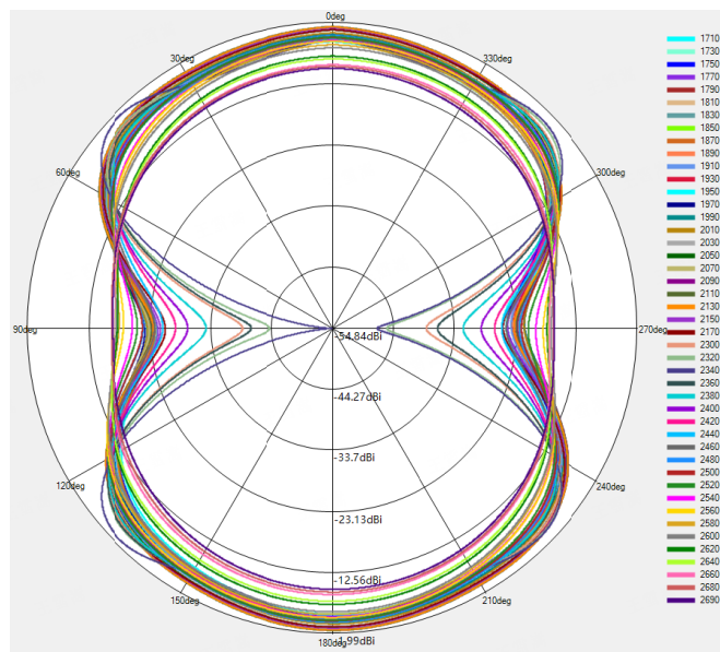
WCDMA B4/LTE B4/B7/B66 NR n7/n66 Phi=0deg
