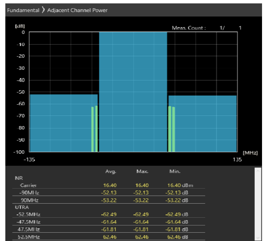
90MHz_30kHz_3655MHz-OFDM QPSK_RB243@0 -52.13,-53.22dB
