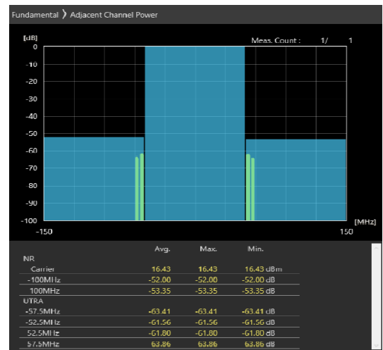
100MHz_30kHz_3650MHz-OFDM QPSK_RB270@0 -52,-53.35dB
