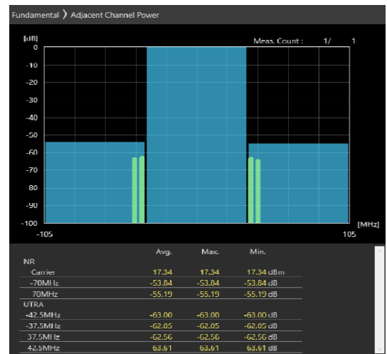
70MHz_30kHz_3665MHz-OFDM QPSK_RB90@45 -53.84,-55.19dB
