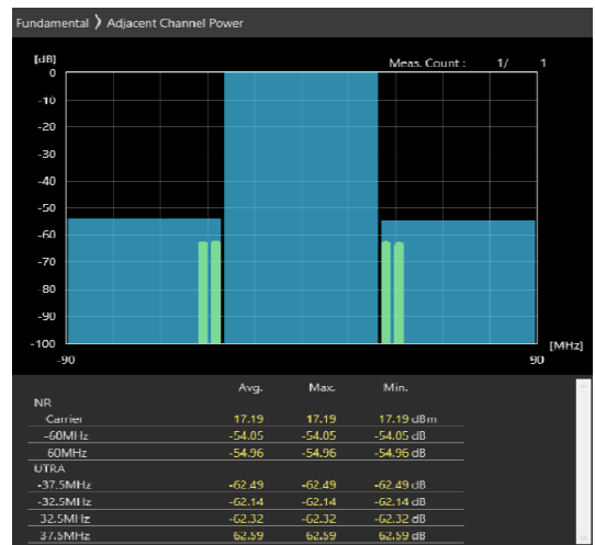
60MHz_30kHz_3670MHz-OFDM QPSK_RB81@40 -54.05,-54.96dB
