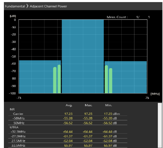
50MHz_30kHz_3675MHz-OFDM QPSK_RB64@32 -55.28,-56.52dB
