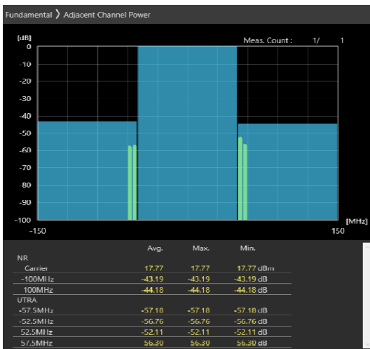
100MHz_30kHz_3650MHz-OFDM QPSK_RB1@272 -43.19,-44.18dB
