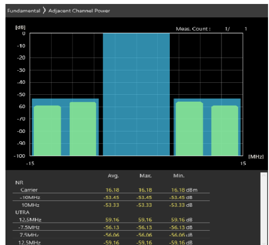
10MHz_30kHz_3695MHz-OFDM QPSK_RB24@0 -53.45,-53.33dB
