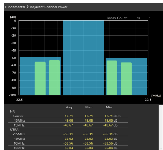
15MHz_30kHz_3692.5MHz-OFDM QPSK_RB36@0 -49.08,-49.67dB
