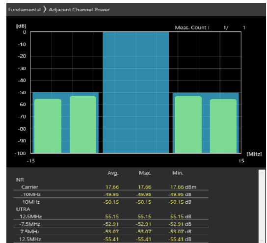
10MHz_30kHz_3695MHz-OFDM QPSK_RB24@0 -49.95,-50.15dB
