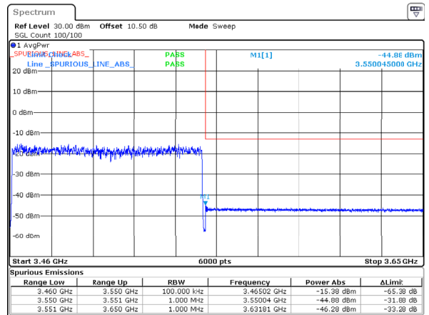
n77_1_90MHz_30kHz_3505MHz_DFT-s-OFDM QPSK_RB243@0
