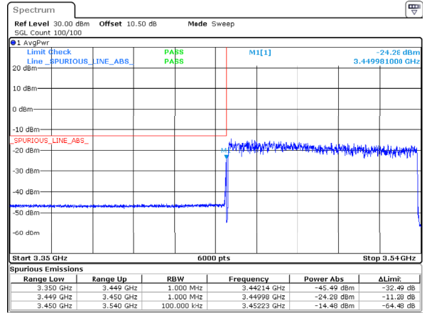
n77_1_90MHz_30kHz_3495MHz_DFT-s-OFDM QPSK_RB243@0
