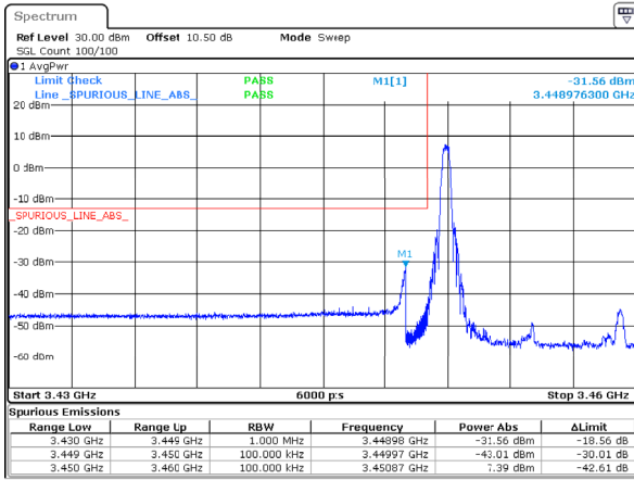
n77_1_10MHz_30kHz_3455MHz_DFT-s-OFDM QPSK_RB1@0
