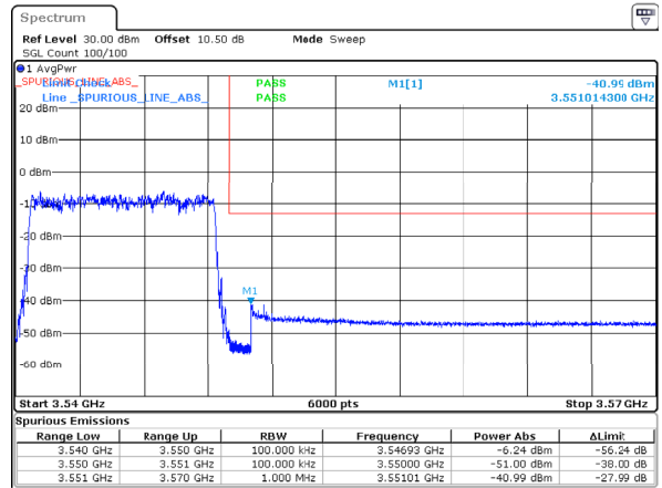
n77_1_10MHz_30kHz_3545MHz_DFT-s-OFDM QPSK_RB24@0
