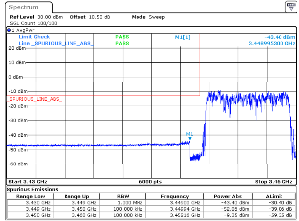
n77_1_10MHz_30kHz_3455MHz_DFT-s-OFDM QPSK_RB24@0
