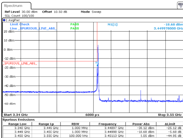
n77_1_100MHz_30kHz_3500MHz_DFT-s-OFDM QPSK_RB1@0
