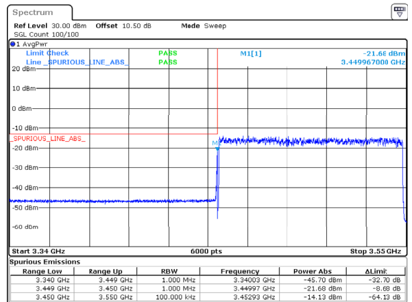
n77_1_100MHz_30kHz_3500MHz_DFT-s-OFDM QPSK_RB270@0
