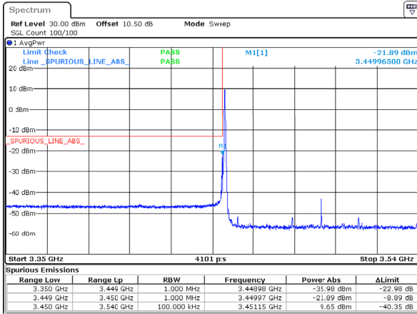
n77_1_90MHz_30kHz_3495MHz_DFT-s-OFDM QPSK_RB1@0
