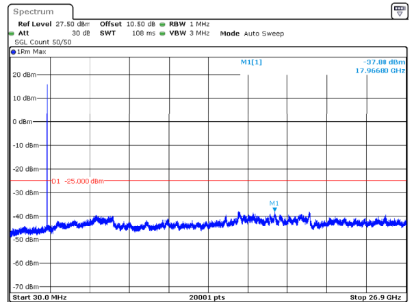
n41_10MHz_30kHz_2501.01MHz_DFT-s-OFDM QPSK_RB24@0 -37.88dBm
