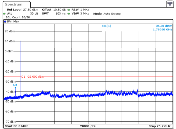
n7_5MHz_15kHz_2502.5MHz_DFT-s-OFDM QPSK_RB1@24 -36.88dBm
