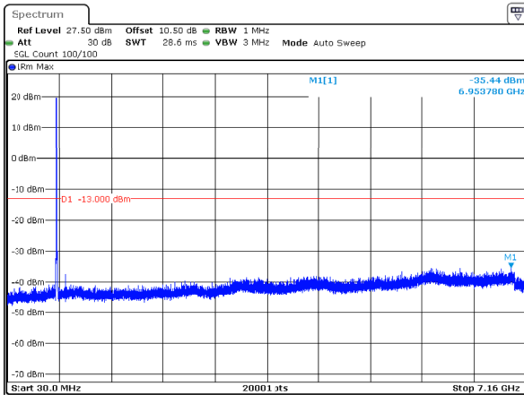
n12_5MHz_15kHz_701.5MHz_DFT-s-OFDM QPSK_RB25@0 -35.44dBm
