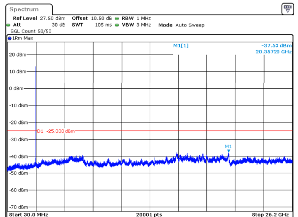
n38_10MHz_30kHz_2575MHz_DFT-s-OFDM QPSK_RB24@0 -37.53dBm
