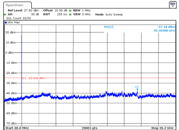
n38_10MHz_30kHz_2575MHz_DFT-s-OFDM QPSK_RB1@0 -37.18dBm
