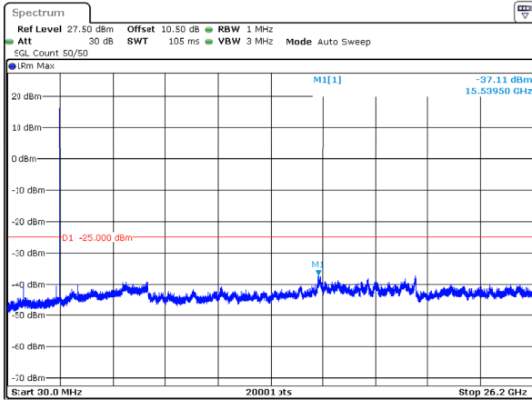
n38_5MHz_15kHz_2617.5MHz_DFT-s-OFDM QPSK_RB1@0 -37.11dBm
