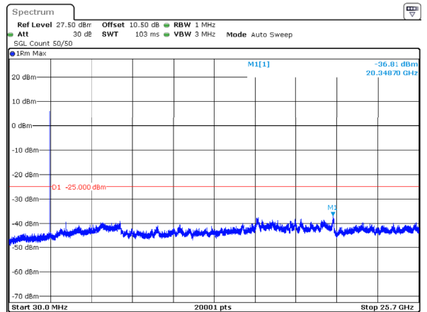
n7_5MHz_15kHz_2535MHz_DFT-s-OFDM QPSK_RB25@0 -36.81dBm
