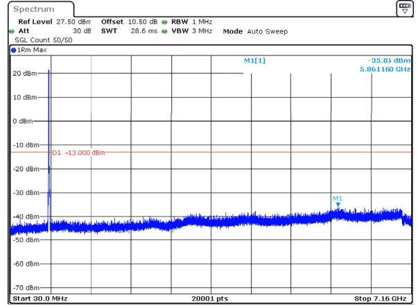
n12_10MHz_15kHz_704MHz_DFT-s-OFDM QPSK_RB50@0 -35.85dBm
