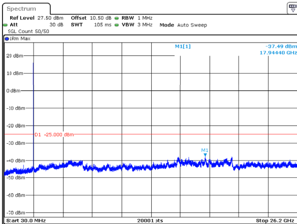
n38_5MHz_15kHz_2617.5MHz_DFT-s-OFDM QPSK_RB25@0 -37.49dBm
