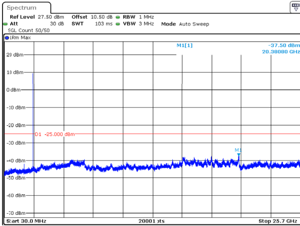
n7_5MHz_15kHz_2502.5MHz_DFT-s-OFDM QPSK_RB1@0 -37.50dBm
