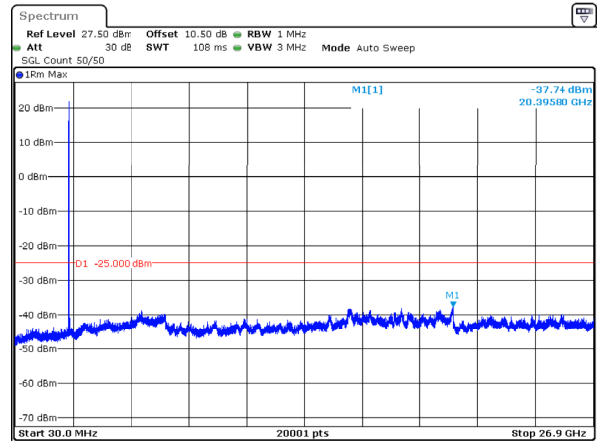
n41_10MHz_30kHz_2501.01MHz_DFT-s-OFDM QPSK_RB1@0 -37.74dBm
