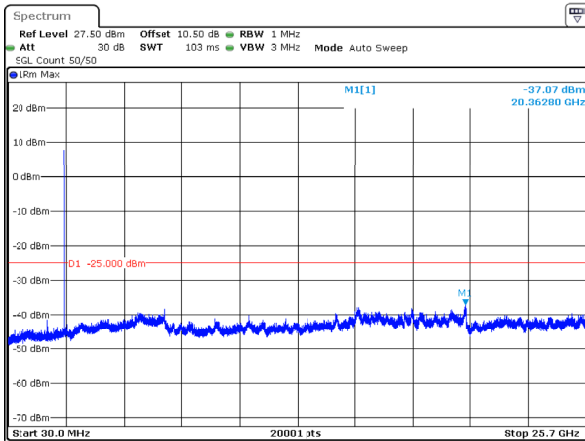
n7_5MHz_15kHz_2502.5MHz_DFT-s-OFDM QPSK_RB25@0 -37.07dBm
