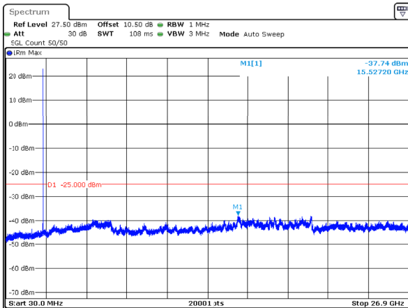
n41_10MHz_30kHz_2501.01MHz_DFT-s-OFDM QPSK_RB1@23 -37.74dBm
