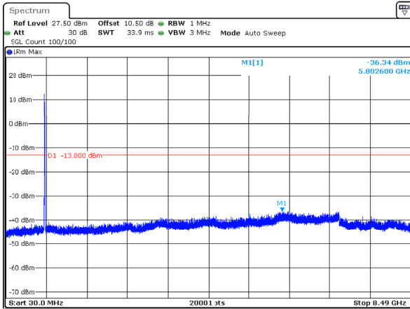
n5_15MHz_15kHz_841.5MHz_DFT-s-OFDM QPSK_RB75@0 -36.34dBm
