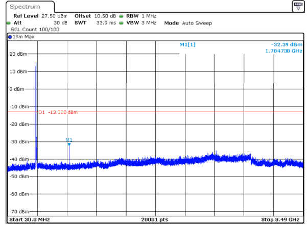
n5_10MHz_15kHz_829MHz_DFT-s-OFDM QPSK_RB50@0 -32.39dBm
