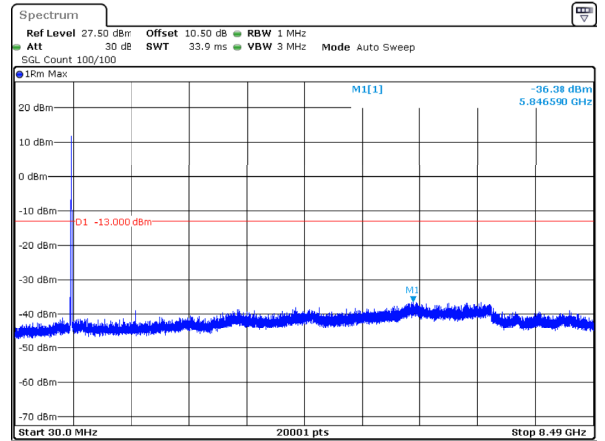
n5_10MHz_15kHz_844MHz_DFT-s-OFDM QPSK_RB50@0 -36.38dBm
