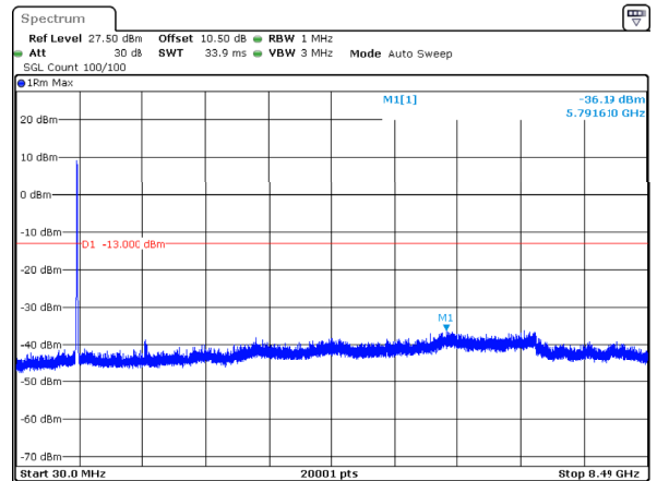
n5_20MHz_15kHz_839MHz_DFT-s-OFDM QPSK_RB100@0 -36.19dBm
