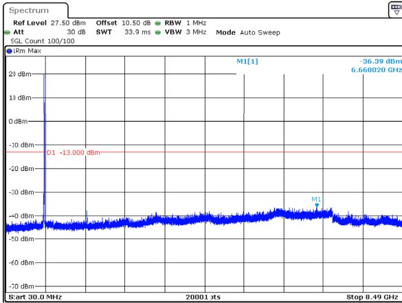
n5_5MHz_15kHz_846.5MHz_DFT-s-OFDM QPSK_RB25@0 -36.39dBm
