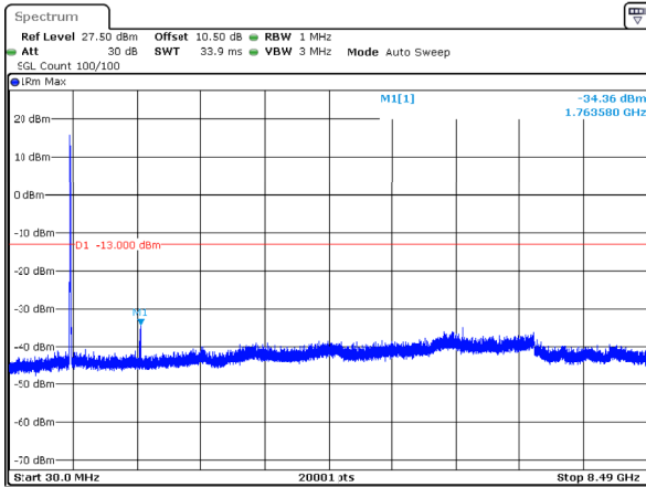
n5_10MHz_15kHz_836.5MHz_DFT-s-OFDM QPSK_RB50@0 -34.36dBm
