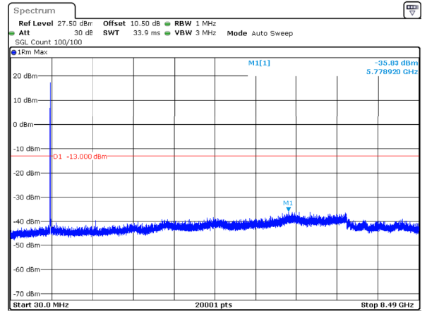
n5_10MHz_15kHz_844MHz_DFT-s-OFDM QPSK_RB1@0 -35.83dBm
