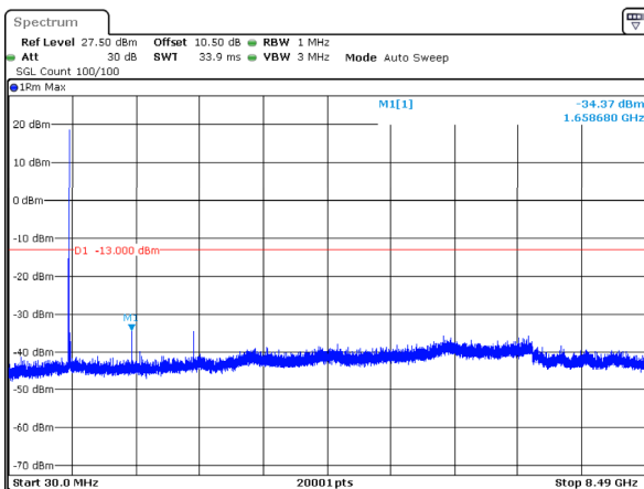
n5_20MHz_15kHz_839MHz_DFT-s-OFDM QPSK_RB1@0 -34.37dBm
