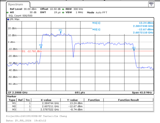
26%OBW Band 41 10MHz/2583.6/Mid QPSK 50@0 Band 41 20MHz/2598.0/Mid QPSK 100@0
